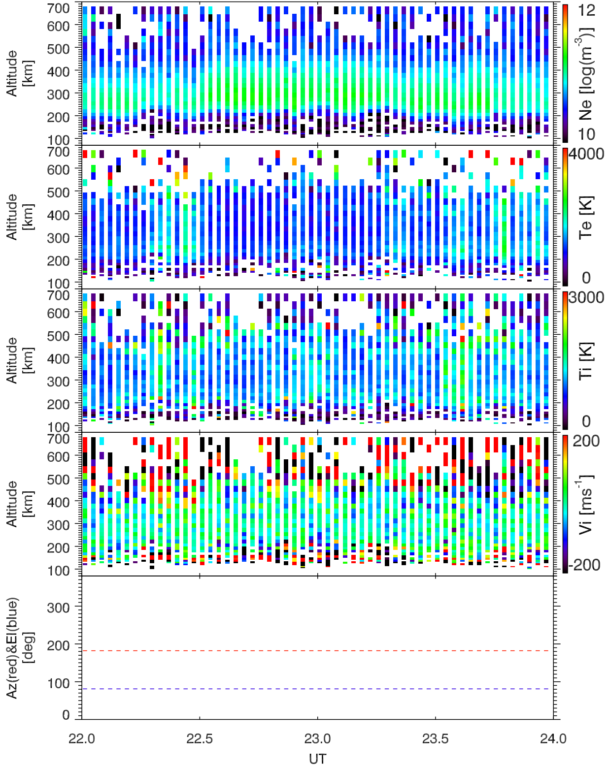
EISCAT 2006-09-21_22_24UT_tau0_ant@42m.
