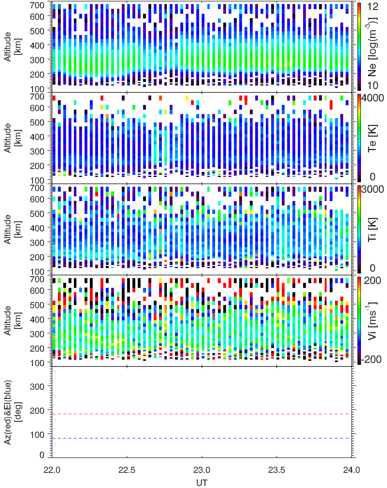
EISCAT 2006-09-22_22_24UT_tau0_ant@42m.
