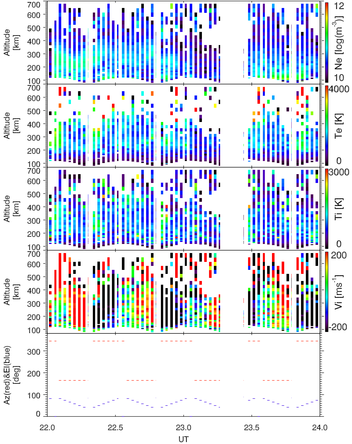
EISCAT 2006-12-13_22_24UT_tau0_ant@32m.
