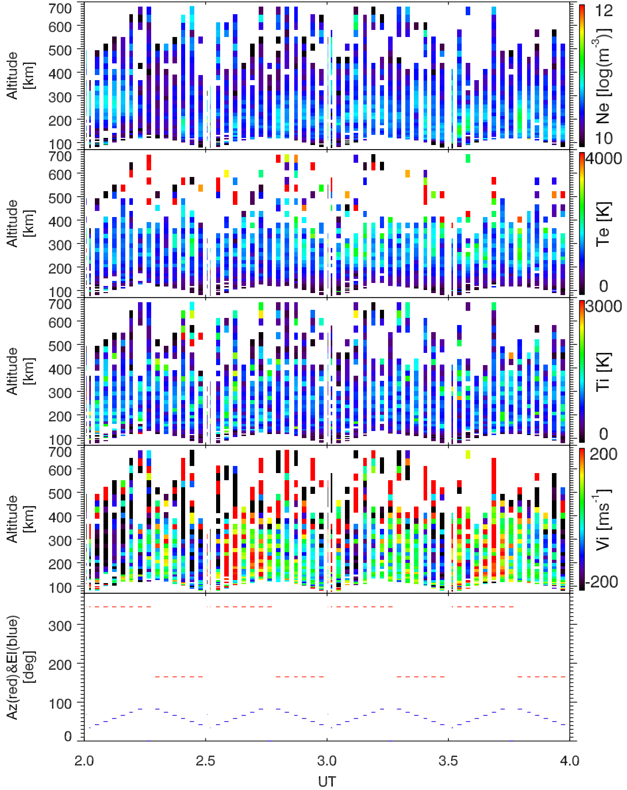
EISCAT 2006-12-17_02_04UT_tau0_ant@32m.
