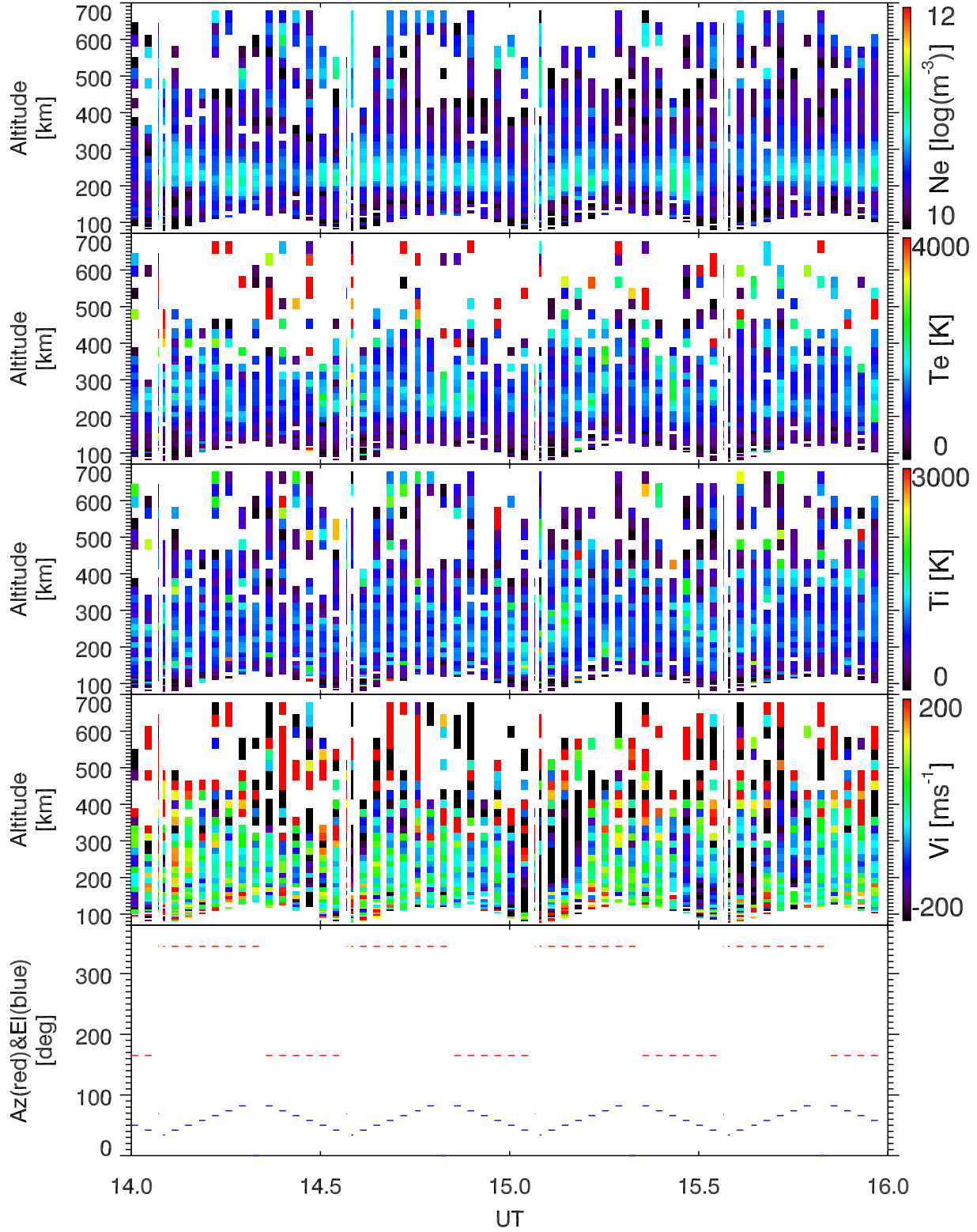
EISCAT 2006-12-17_14_16UT_tau0_ant@32m.
