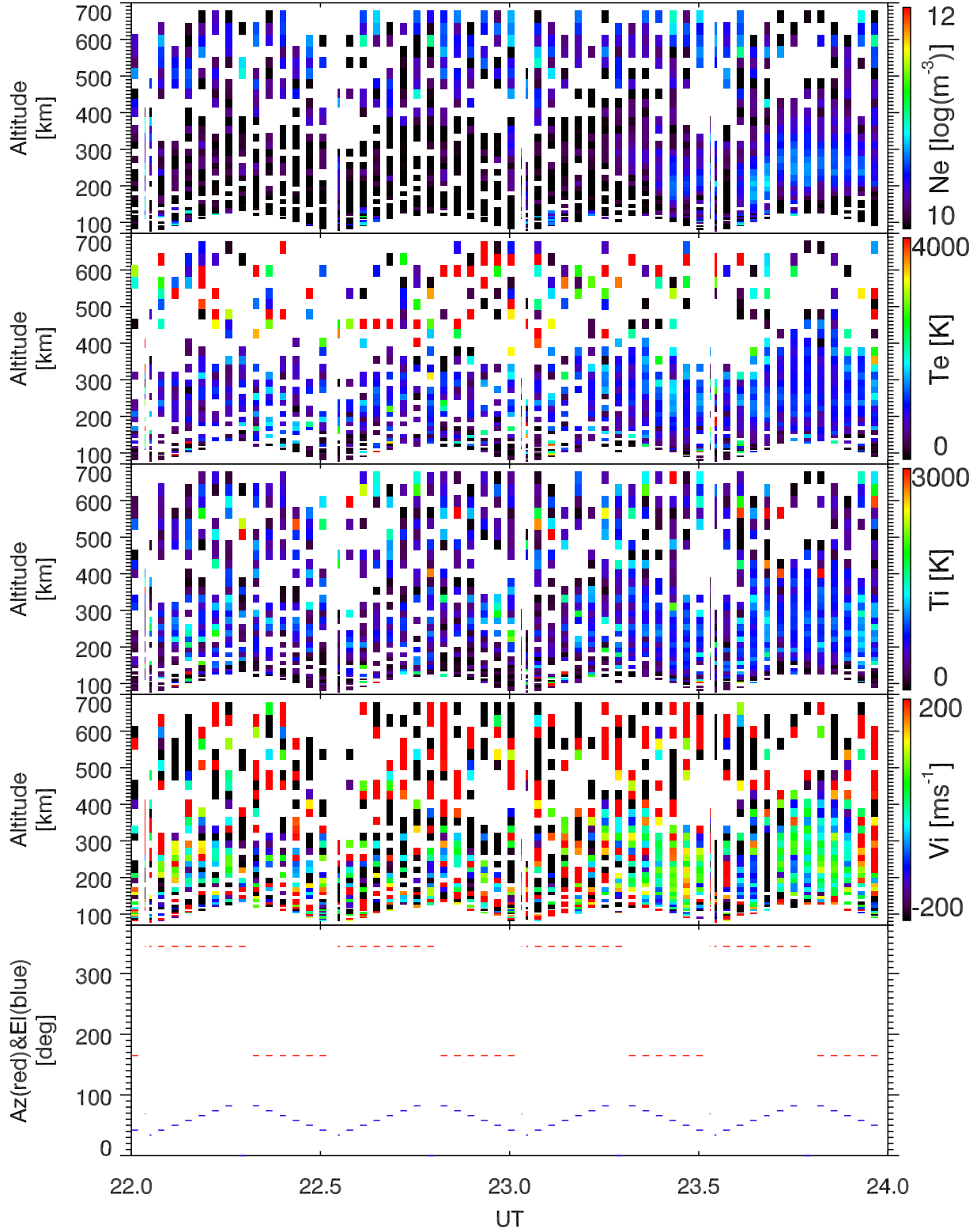
EISCAT 2006-12-17_22_24UT_tau0_ant@32m.
