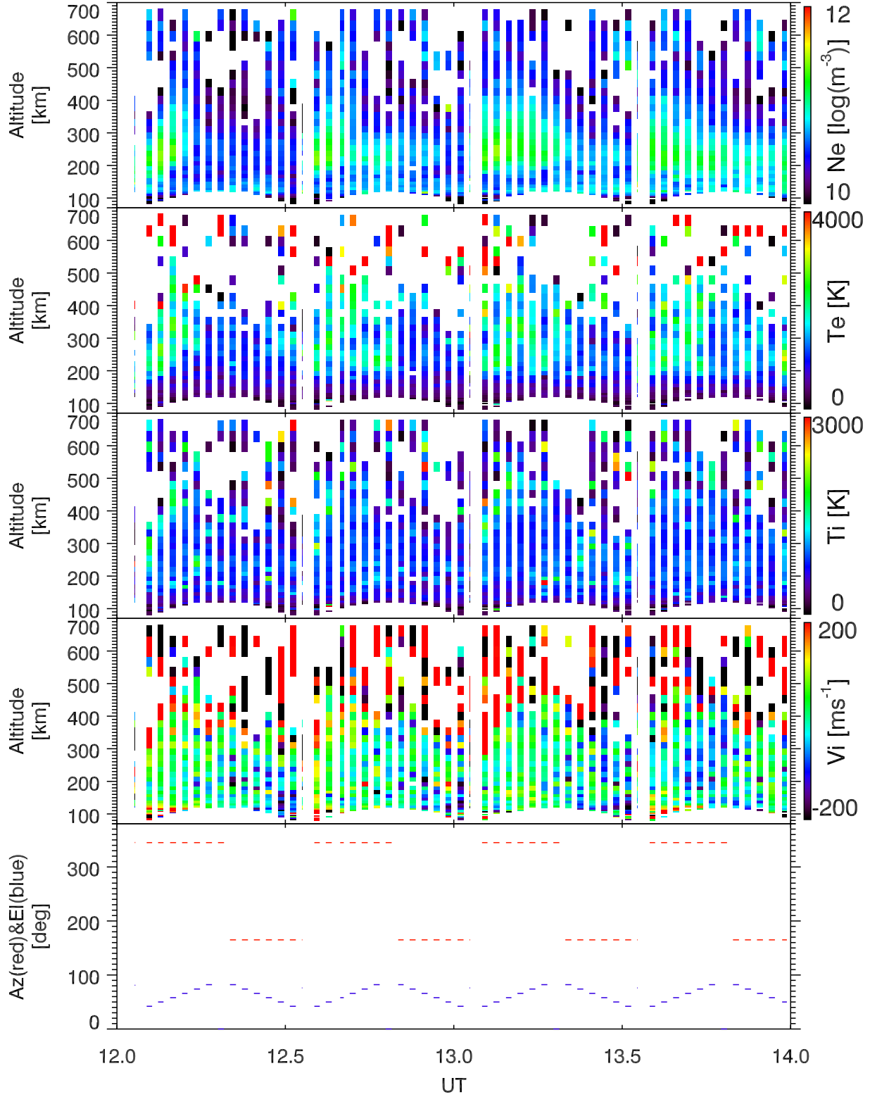
EISCAT 2006-12-18_12_14UT_tau0_ant@32m.
