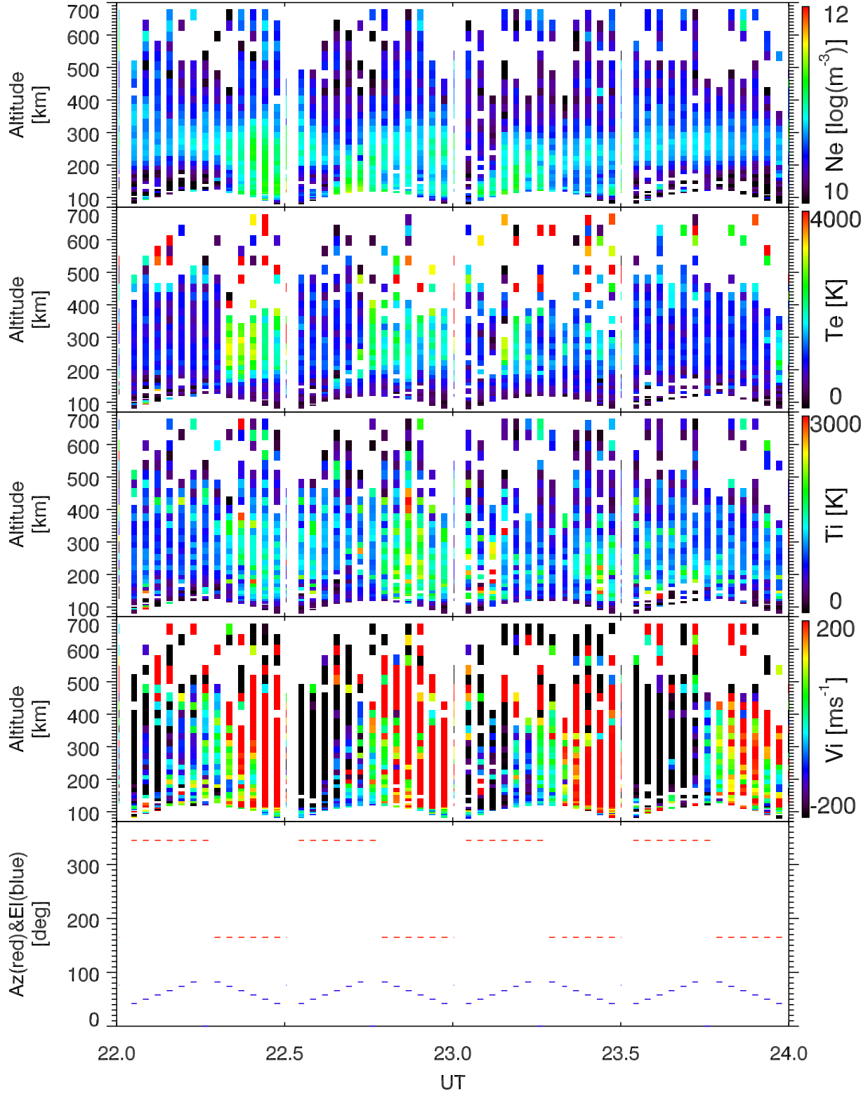
EISCAT 2006-12-18_22_24UT_tau0_ant@32m.
