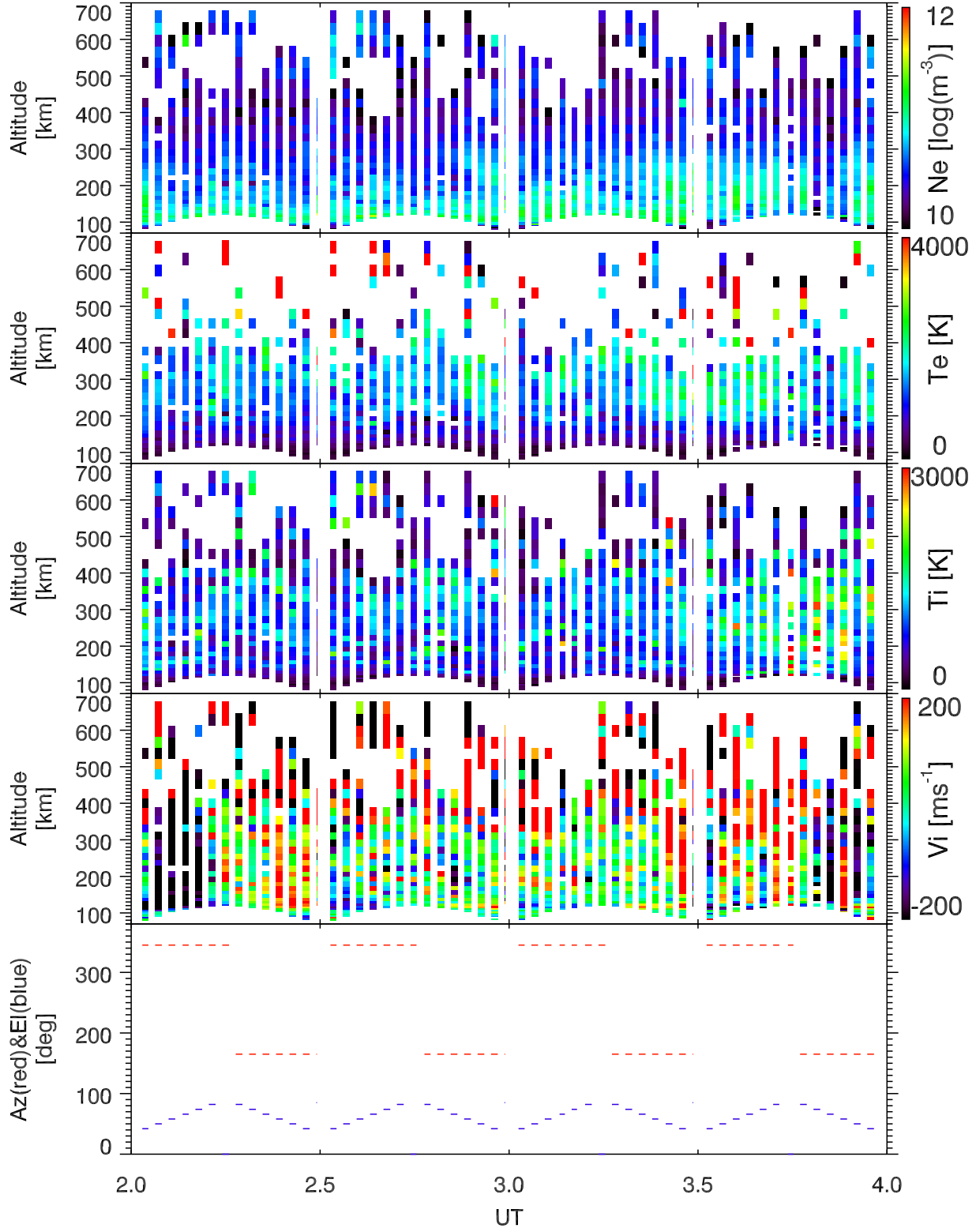
EISCAT 2006-12-20_02_04UT_tau0_ant@32m.
