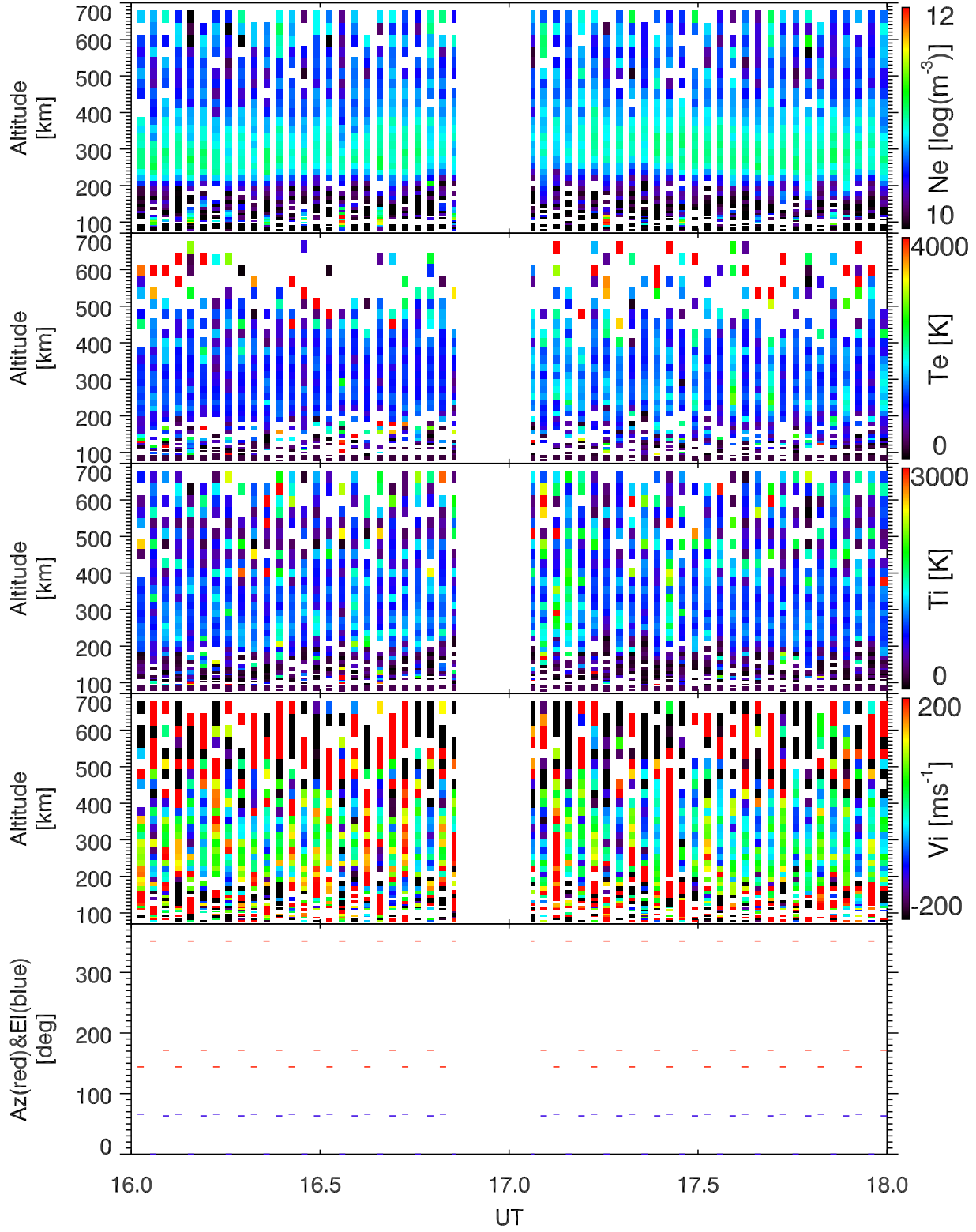
EISCAT 2007-02-08_16_18UT_steffe_ant@32m.
