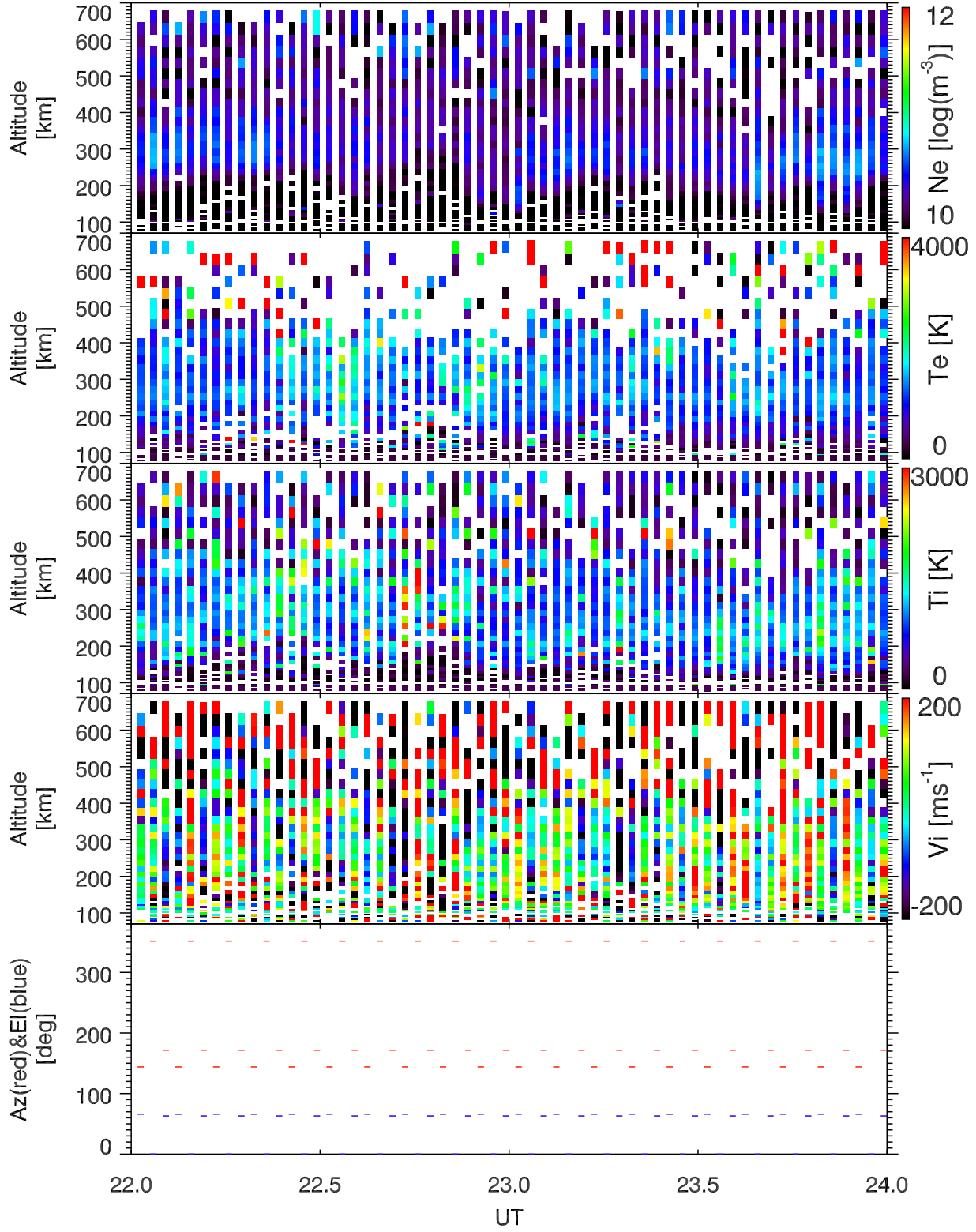
EISCAT 2007-03-01_22_24UT_steffe_ant@32m.
