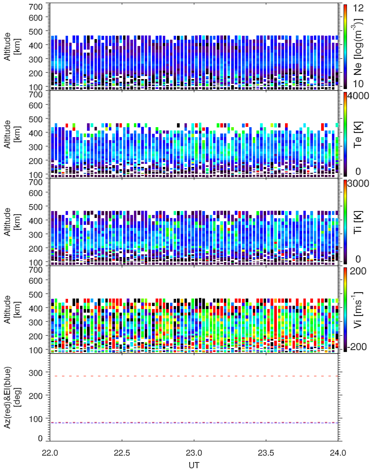
EISCAT 2007-03-20_22_24UT_ipy_ant@32m.
