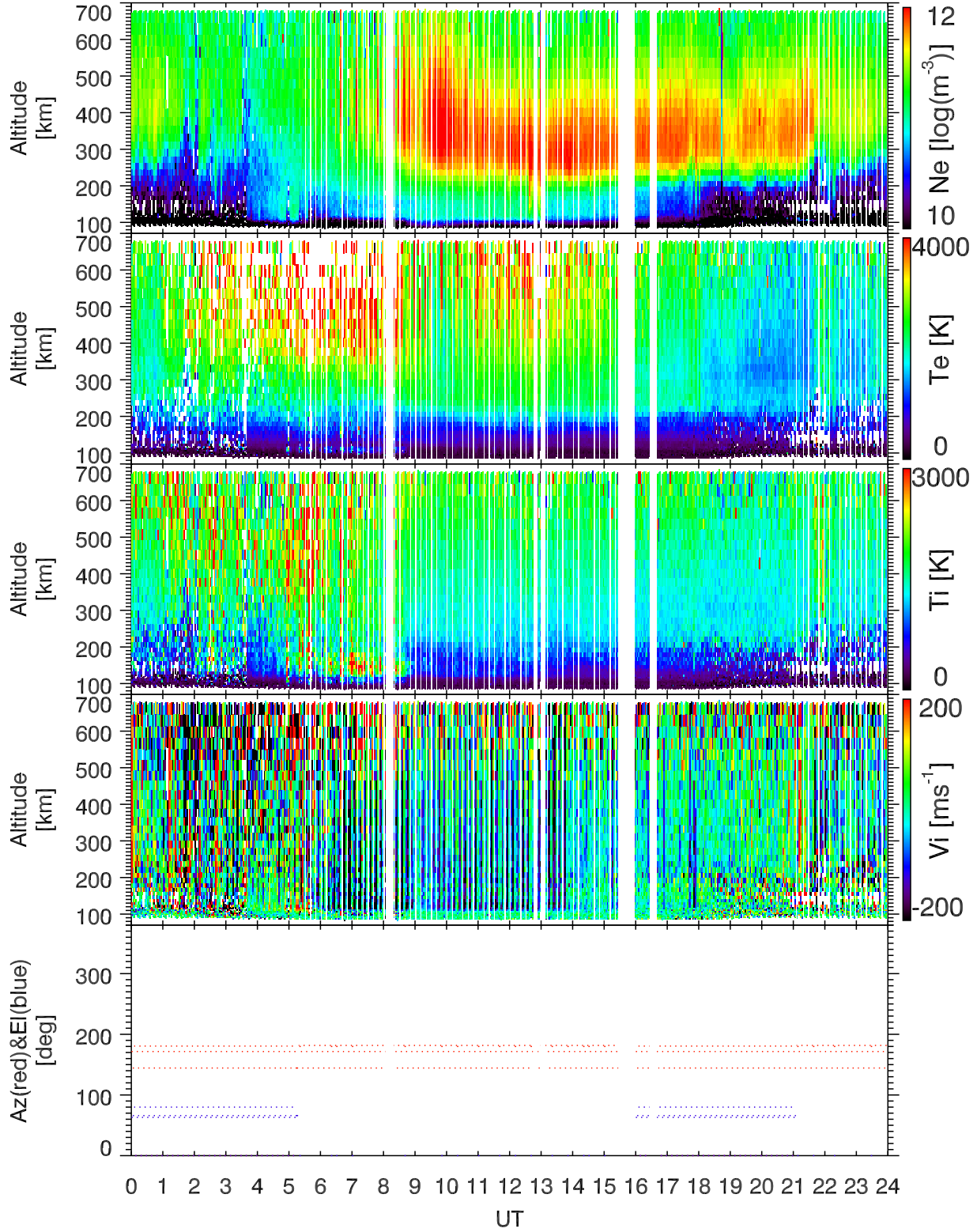
EISCAT 2000-03-19_00_24UT_gup3c_ant@32m.
