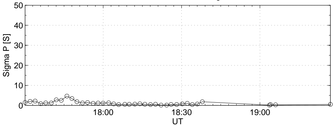
2004-09-21 tau0@42m Sigma P
