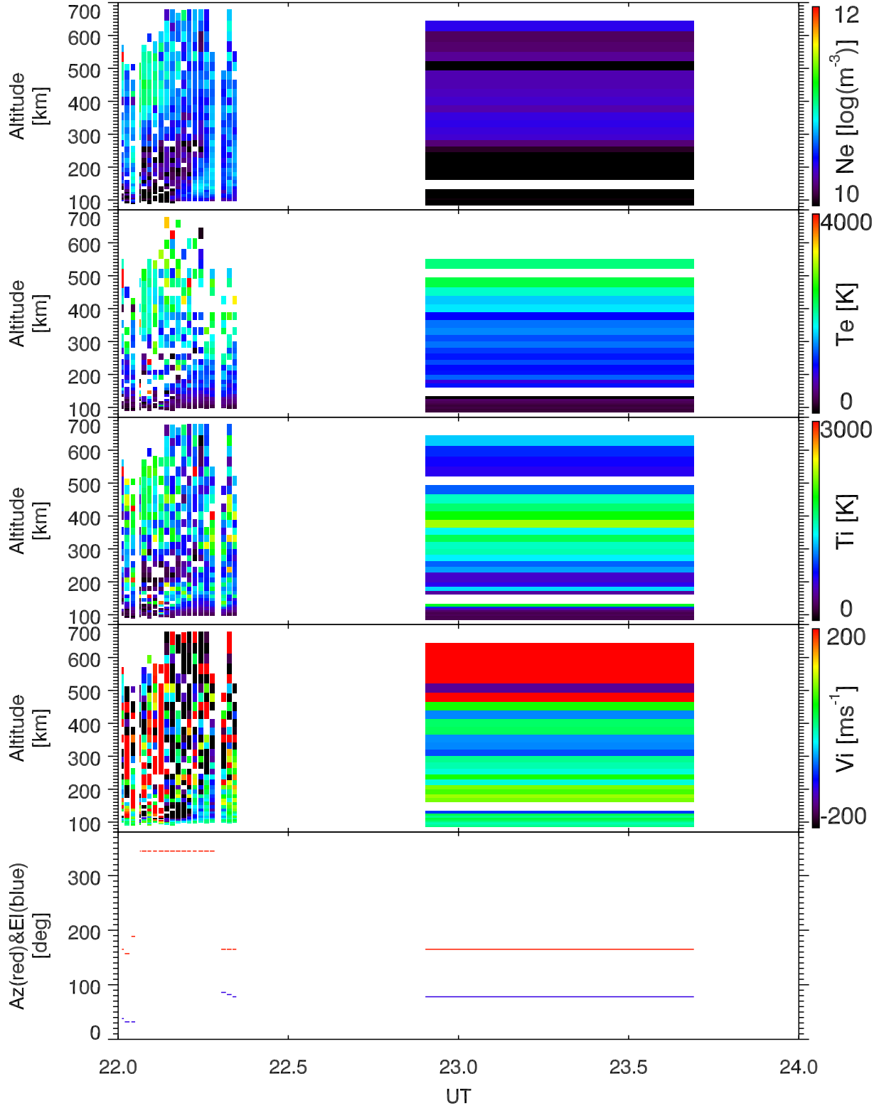
EISCAT 1998-10-19_22_24UT_gup3c_ant@32m.
