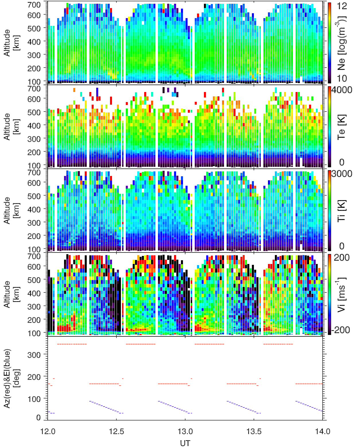
EISCAT 1999-04-21_12_14UT_gup3c_ant@32m.
