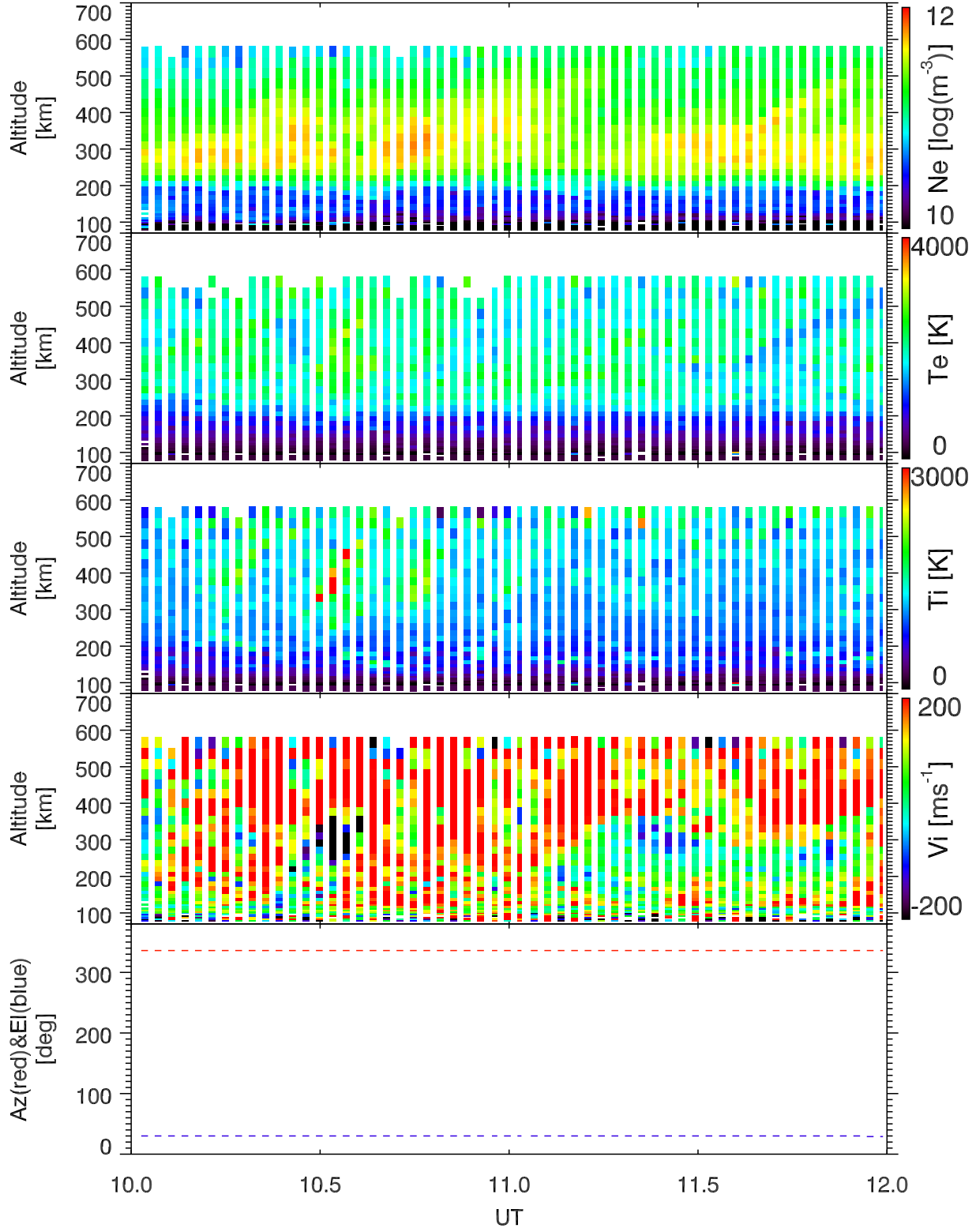
EISCAT 2001-02-18_10_12UT_tau0_ant@32m.
