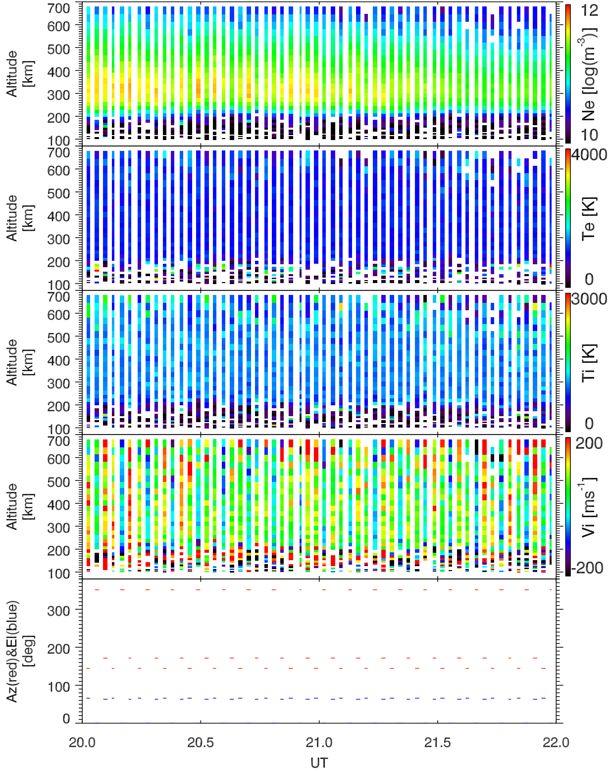
EISCAT 2001-02-18_20_22UT_tau0_ant@32m.
