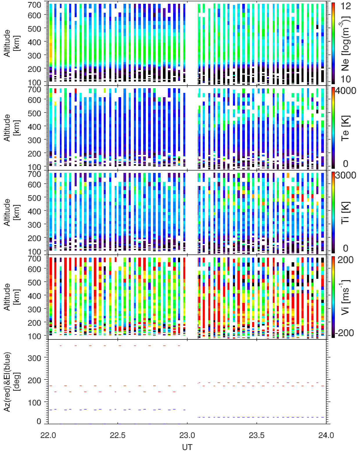
EISCAT 2001-02-19_22_24UT_tau0_ant@32m.
