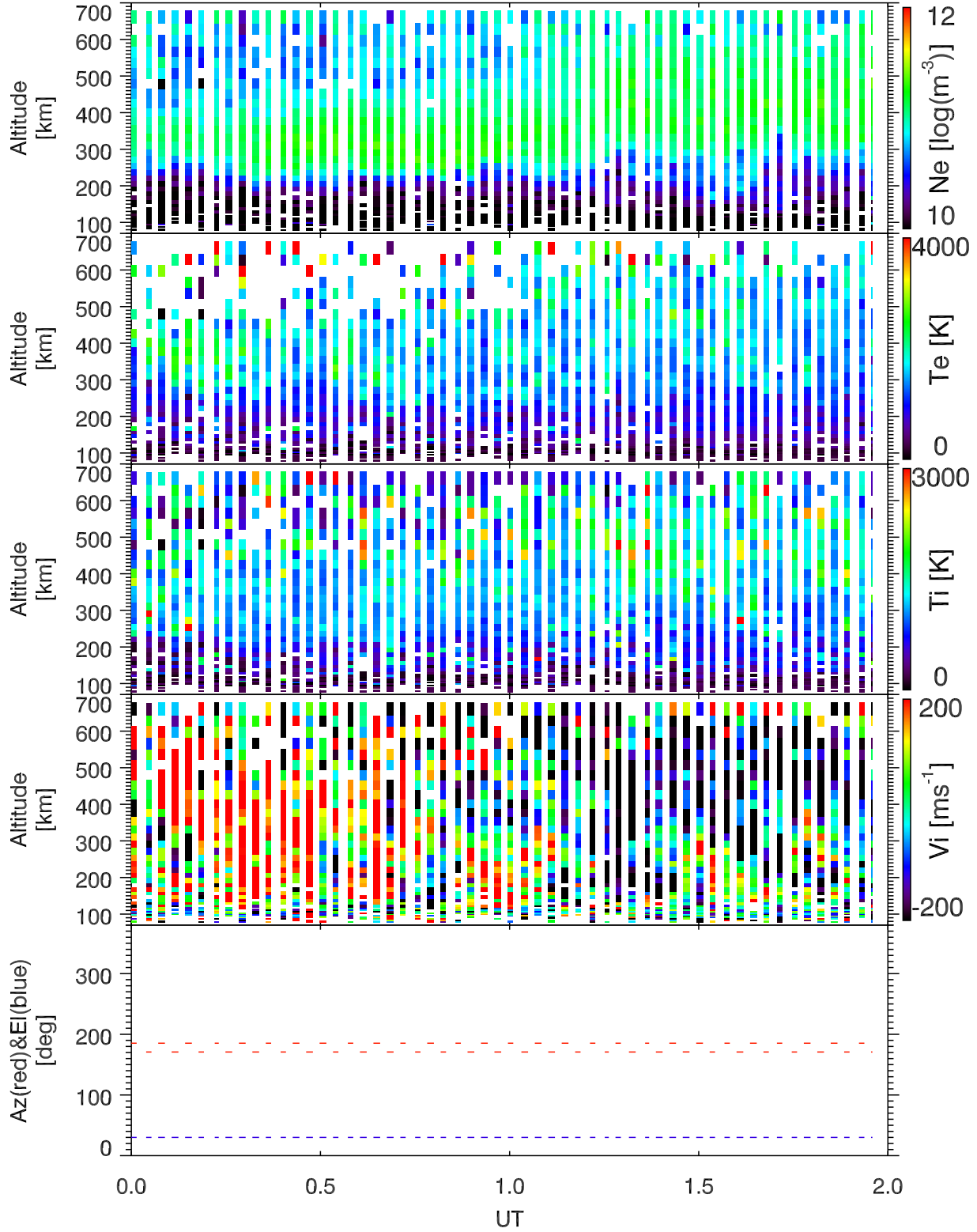
EISCAT 2001-02-20_00_02UT_tau0_ant@32m.
