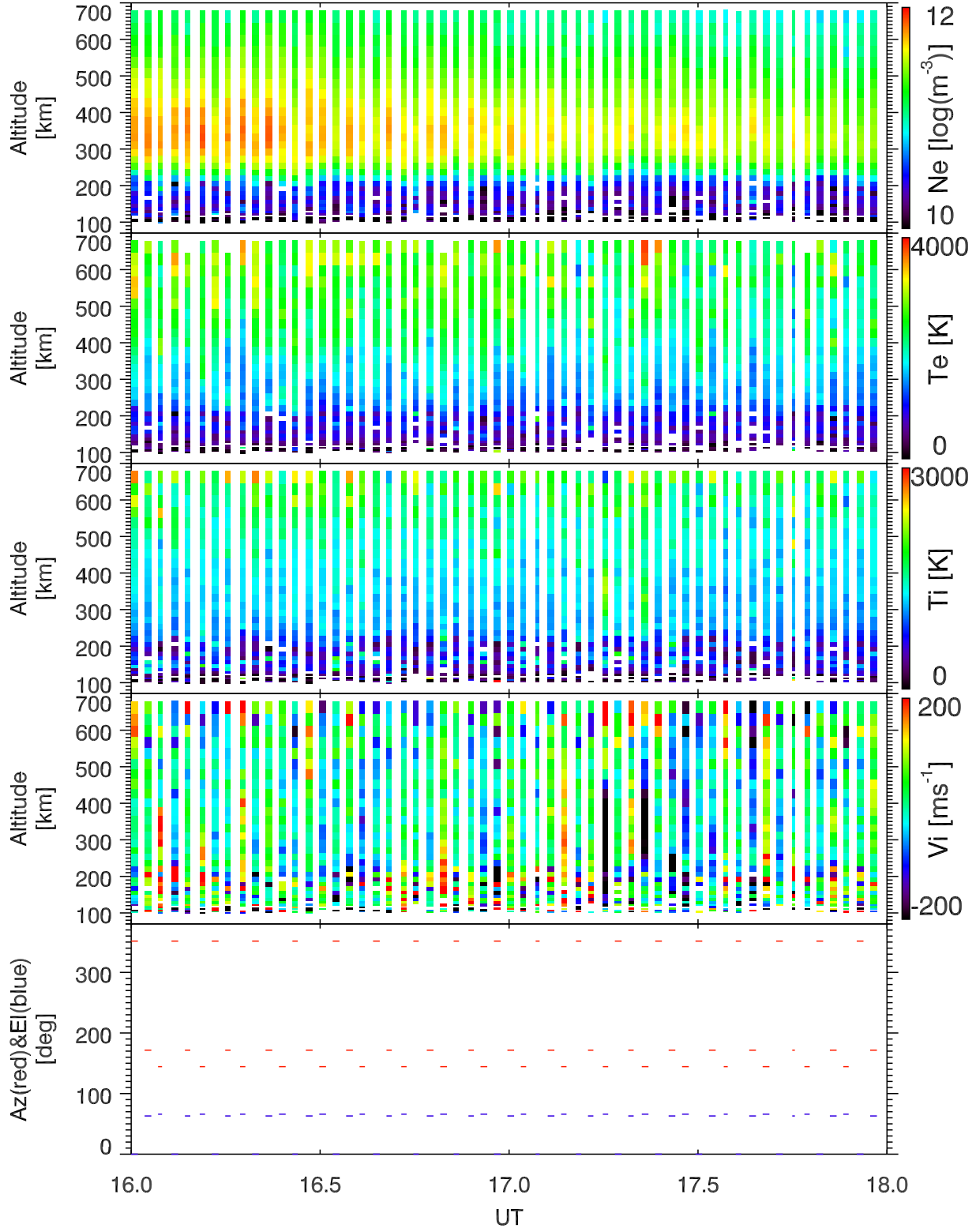
EISCAT 2001-02-20_16_18UT_tau0_ant@32m.
