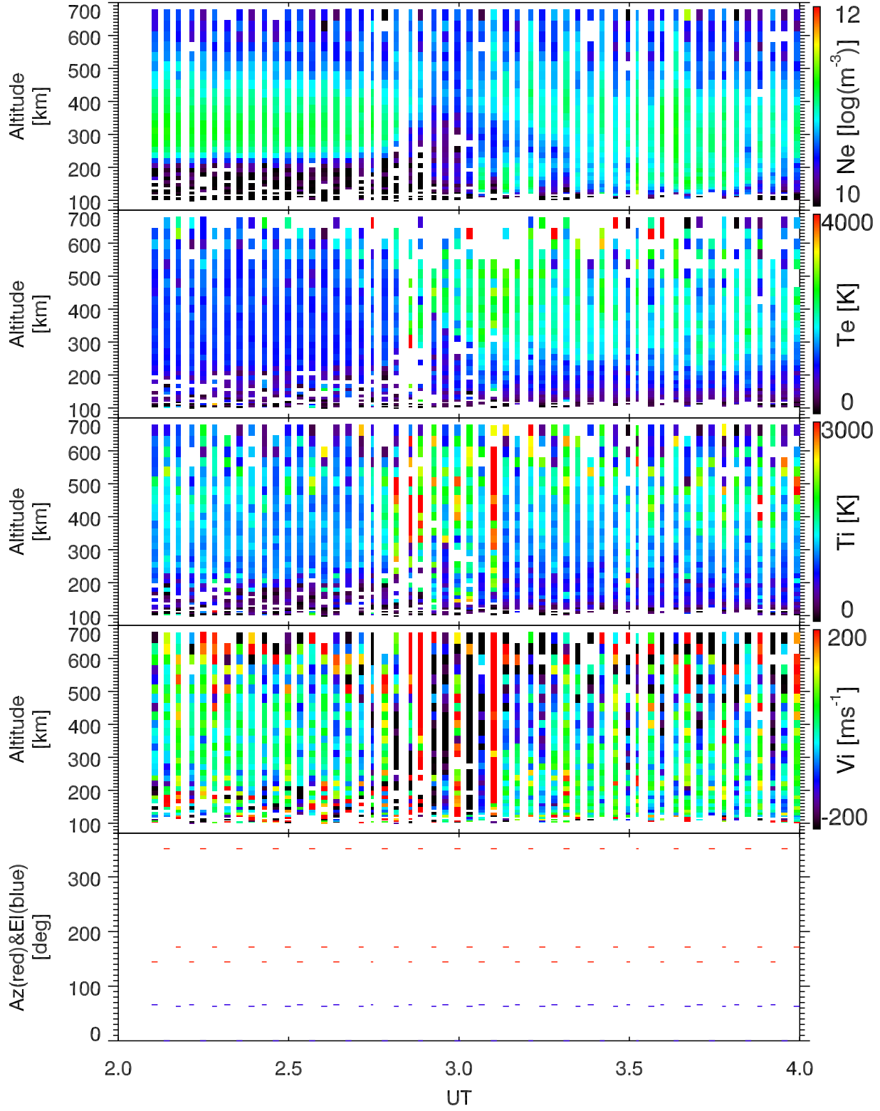
EISCAT 2001-02-21_02_04UT_tau0_ant@32m.
