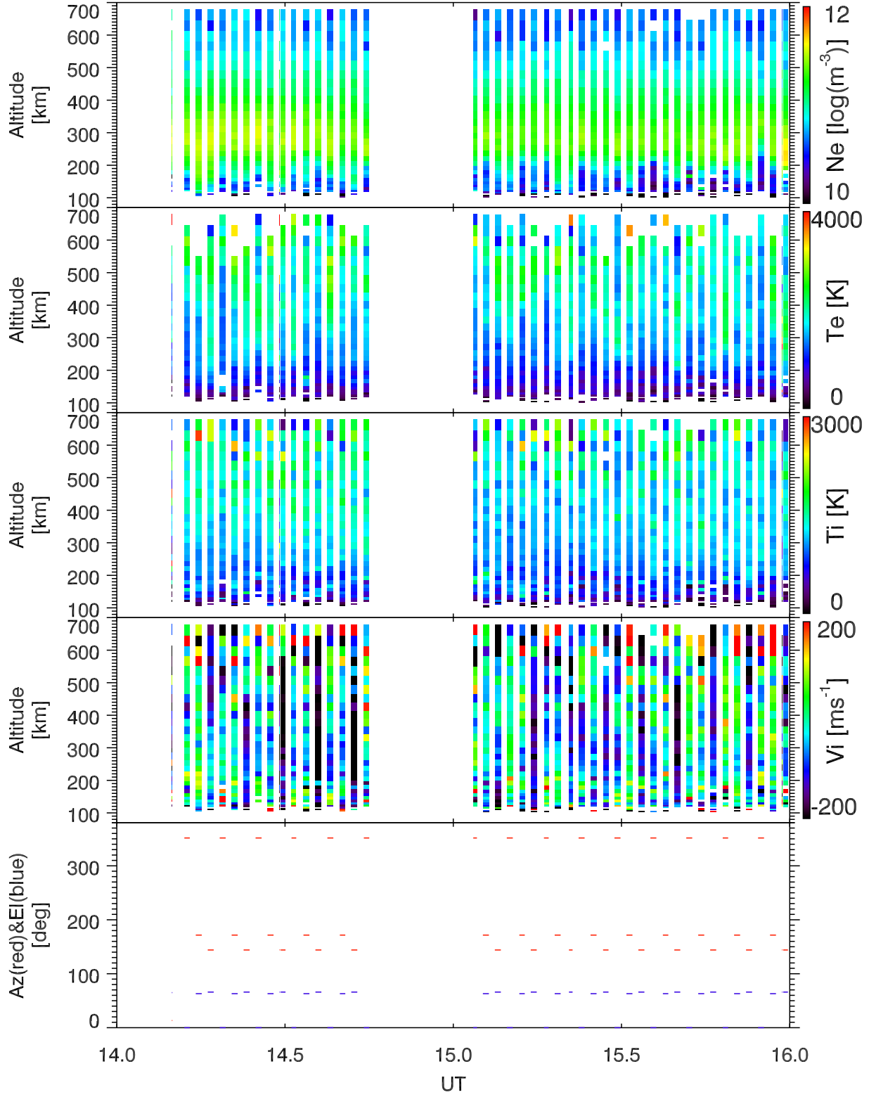
EISCAT 2001-12-11_14_16UT_tau0_ant@32m.
