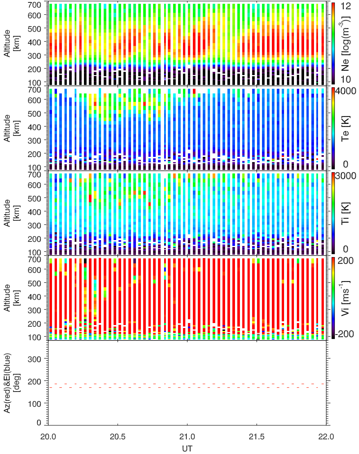
EISCAT 2001-12-12_20_22UT_tau0_ant@32m.
