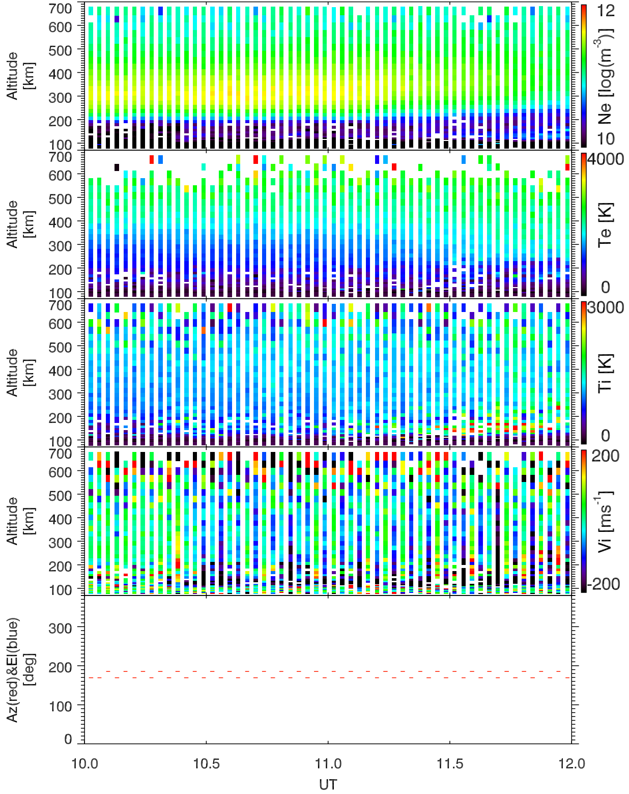
EISCAT 2001-12-14_10_12UT_tau0_ant@32m.
