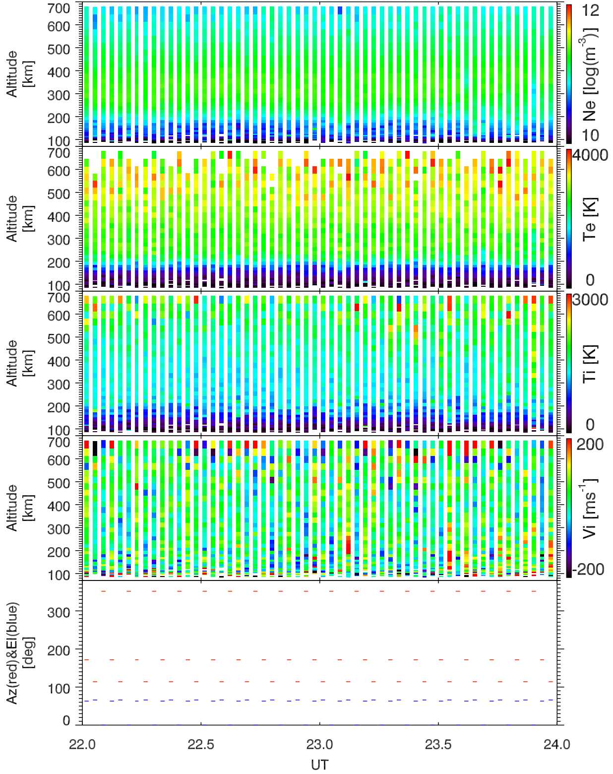
EISCAT 2002-07-28_22_24UT_tau0_ant@32m.
