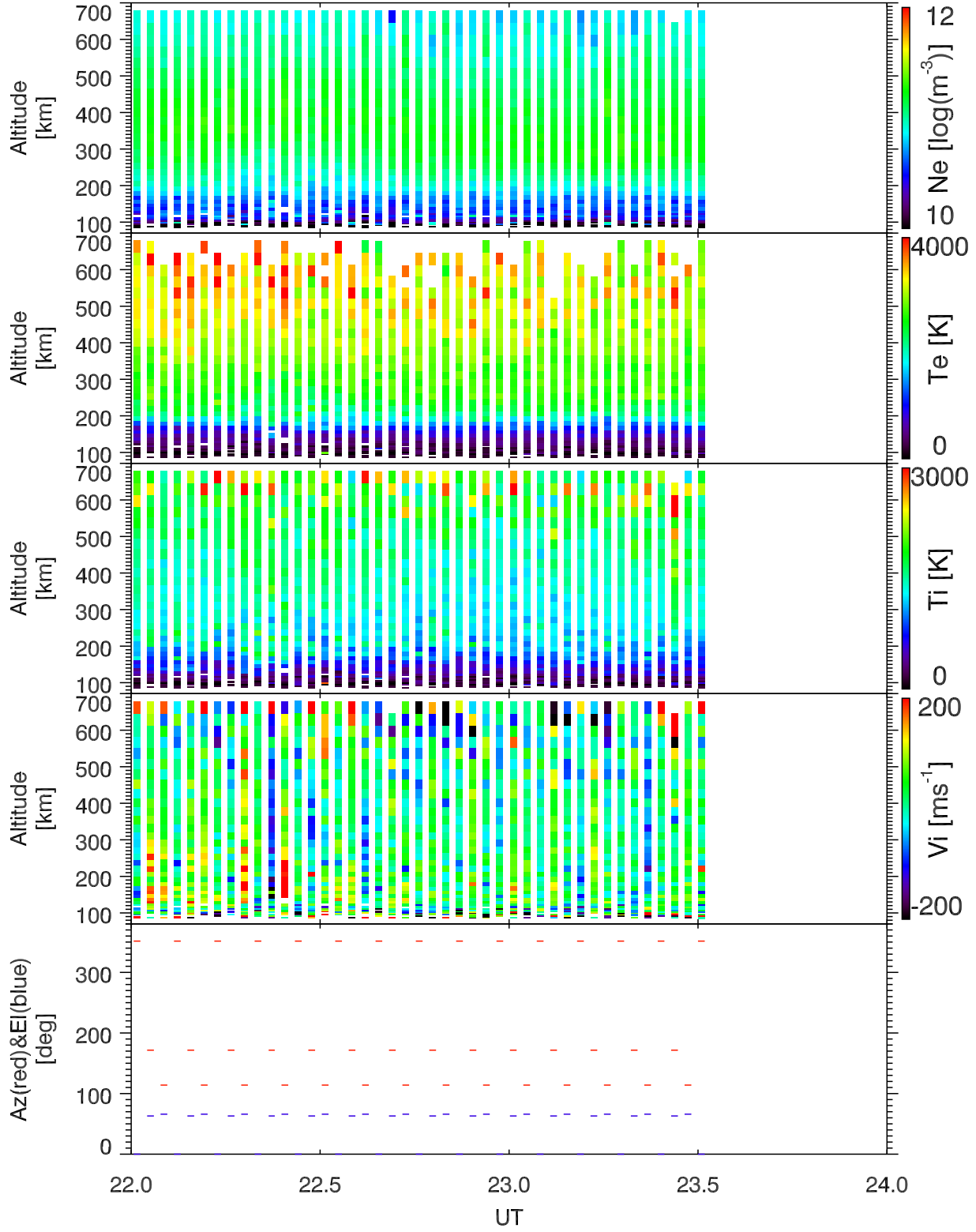
EISCAT 2002-07-29_22_24UT_tau0_ant@32m.
