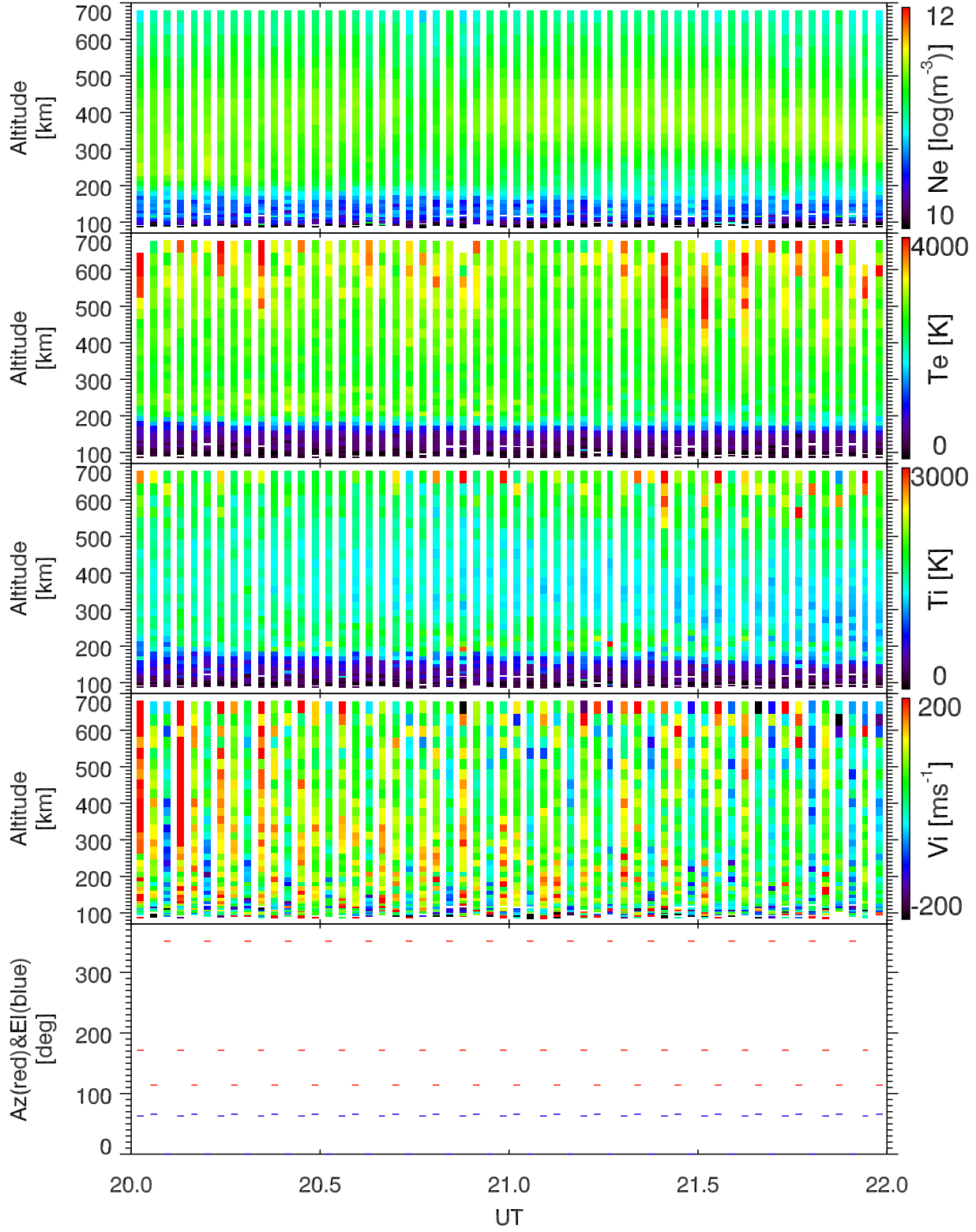
EISCAT 2002-07-30_20_22UT_tau0_ant@32m.
