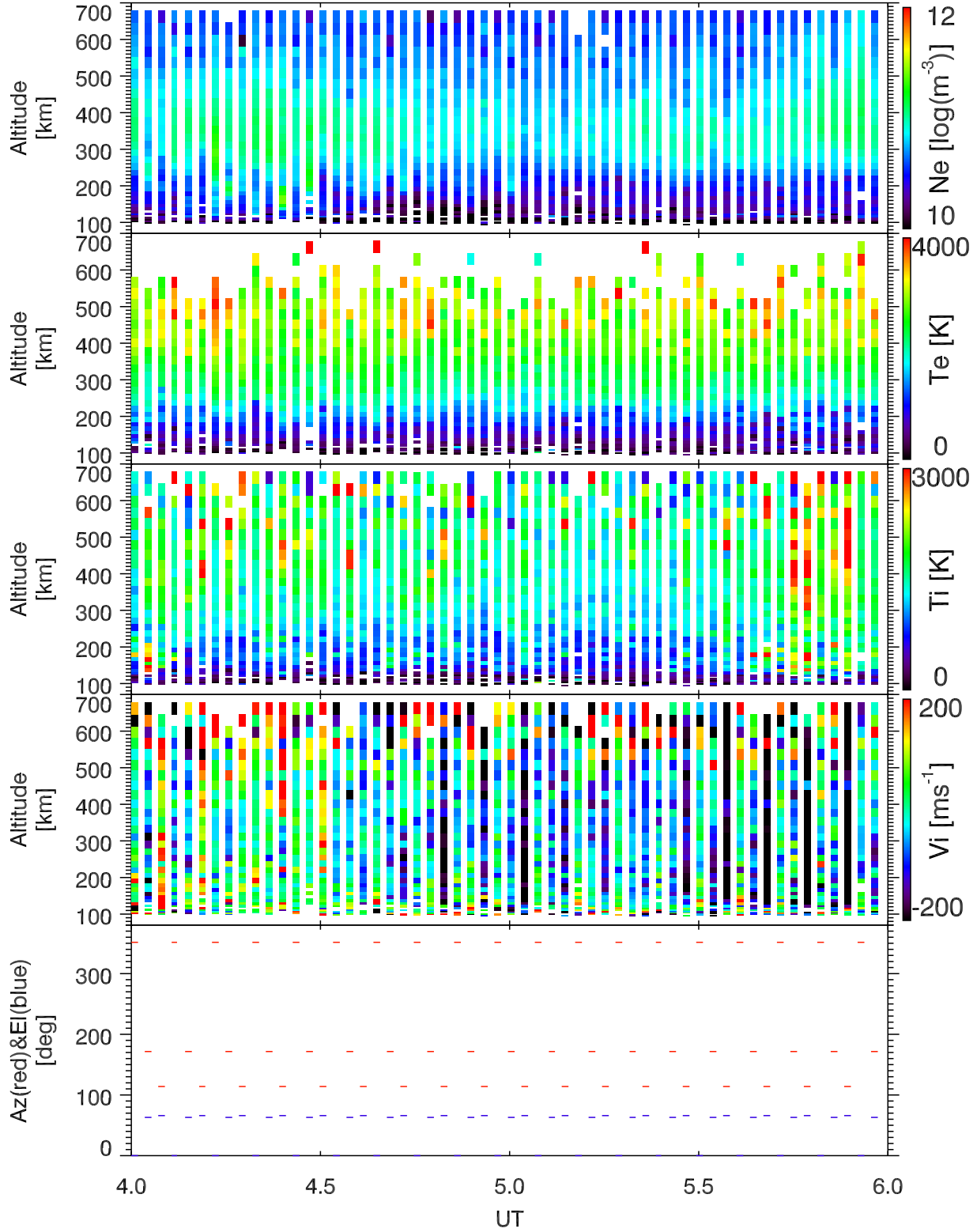
EISCAT 2002-10-06_04_06UT_tau0_ant@32m.
