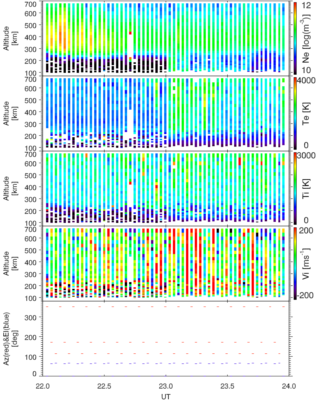
EISCAT 2002-10-17_22_24UT_tau0_ant@32m.
