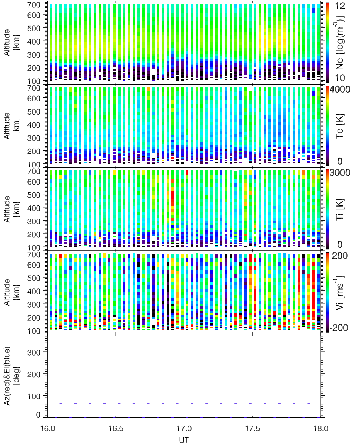
EISCAT 2002-10-18_16_18UT_tau0_ant@32m.
