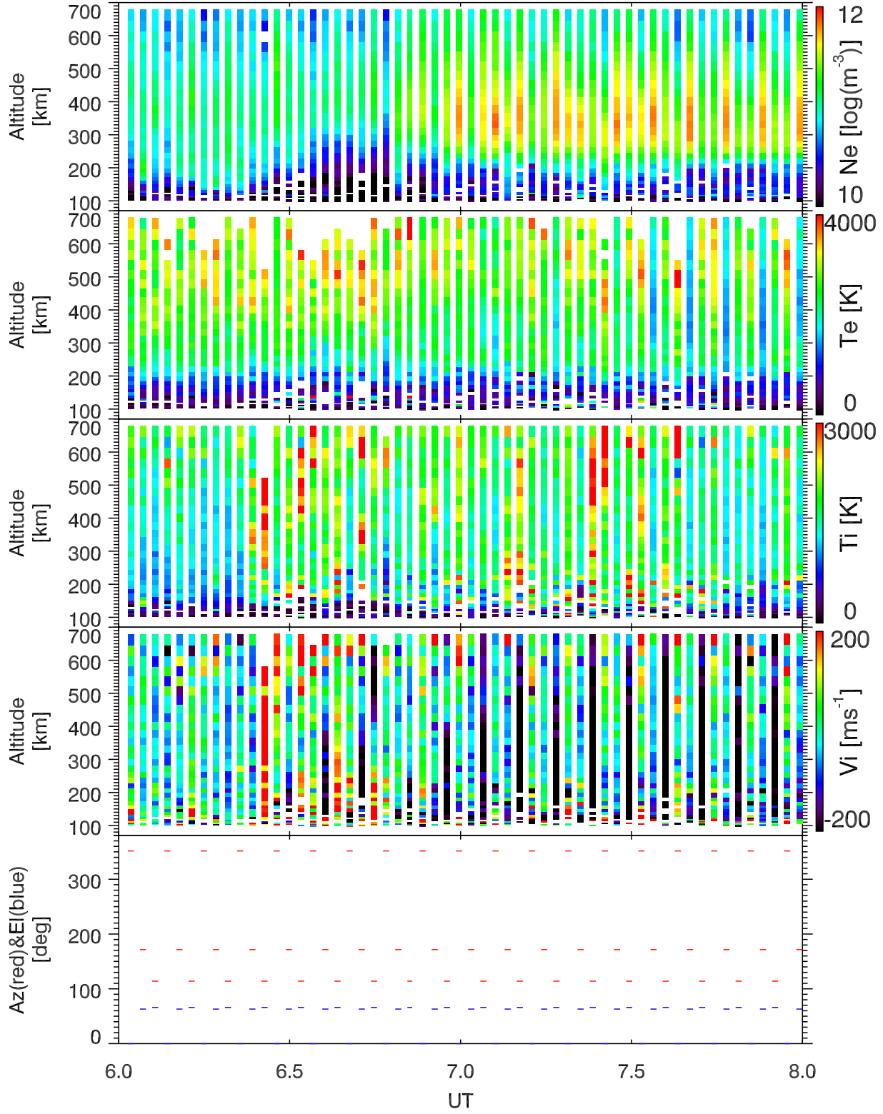
EISCAT 2002-10-26_06_08UT_tau0_ant@32m.
