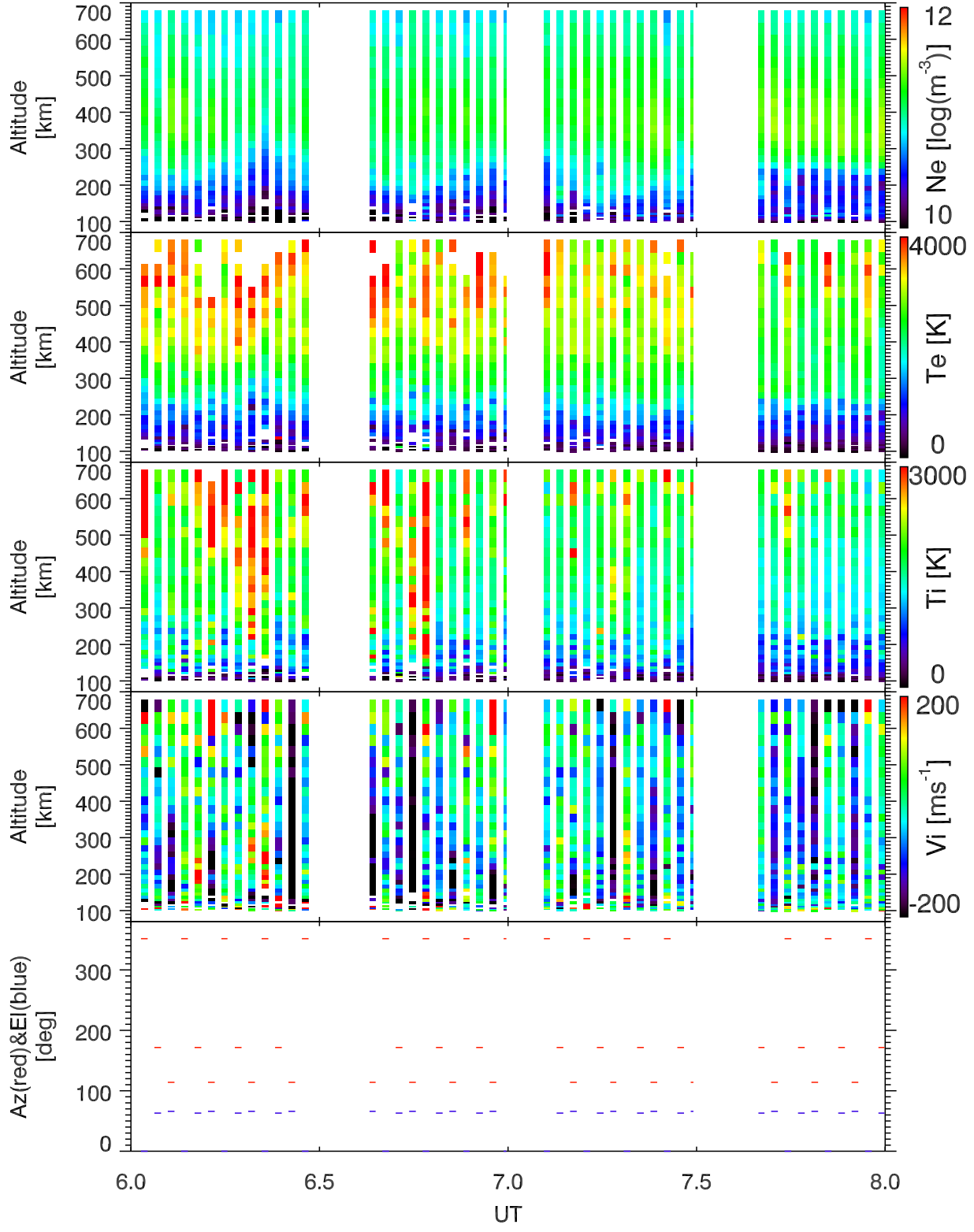
EISCAT 2002-10-28_06_08UT_tau0_ant@32m.
