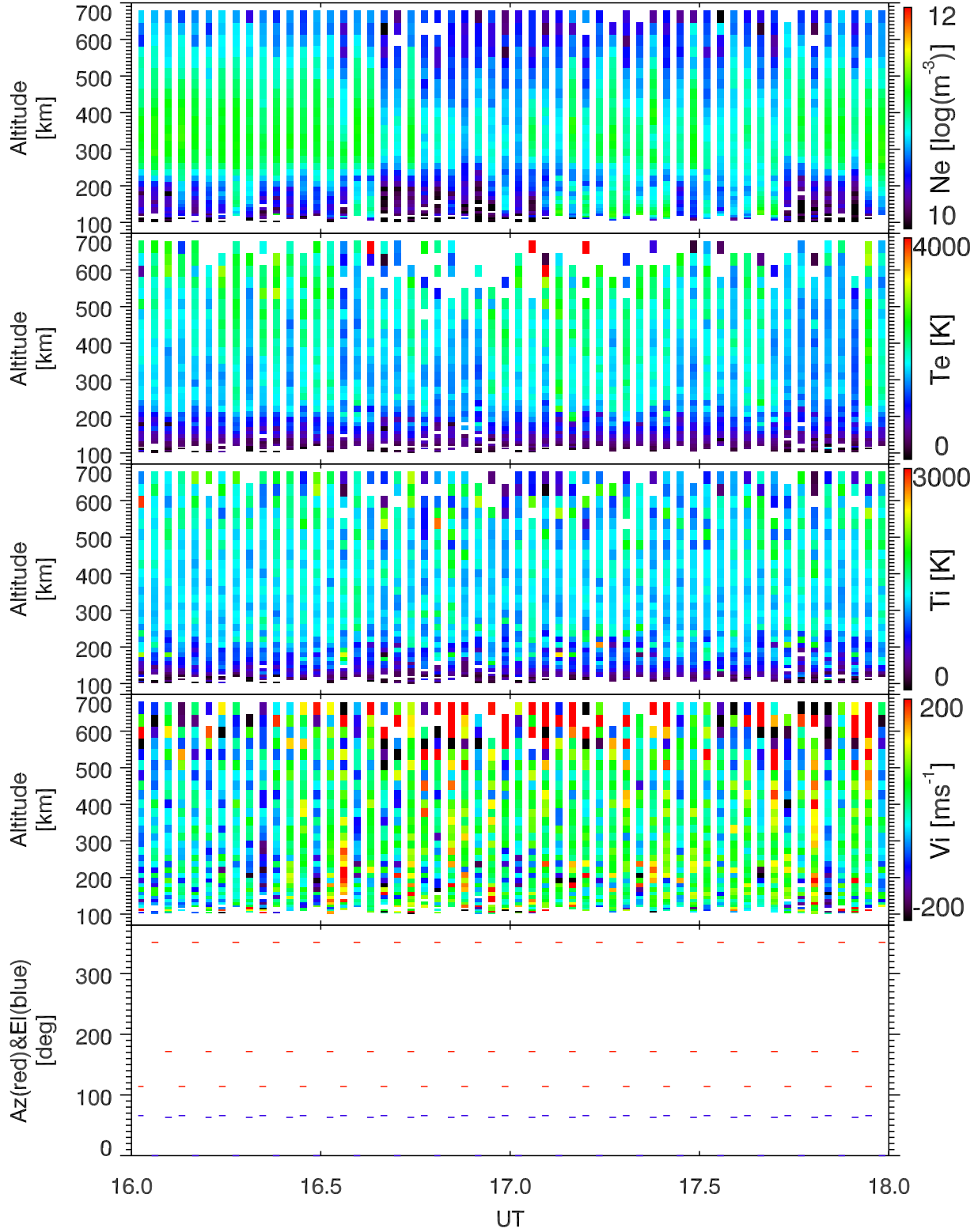
EISCAT 2002-10-28_16_18UT_tau0_ant@32m.
