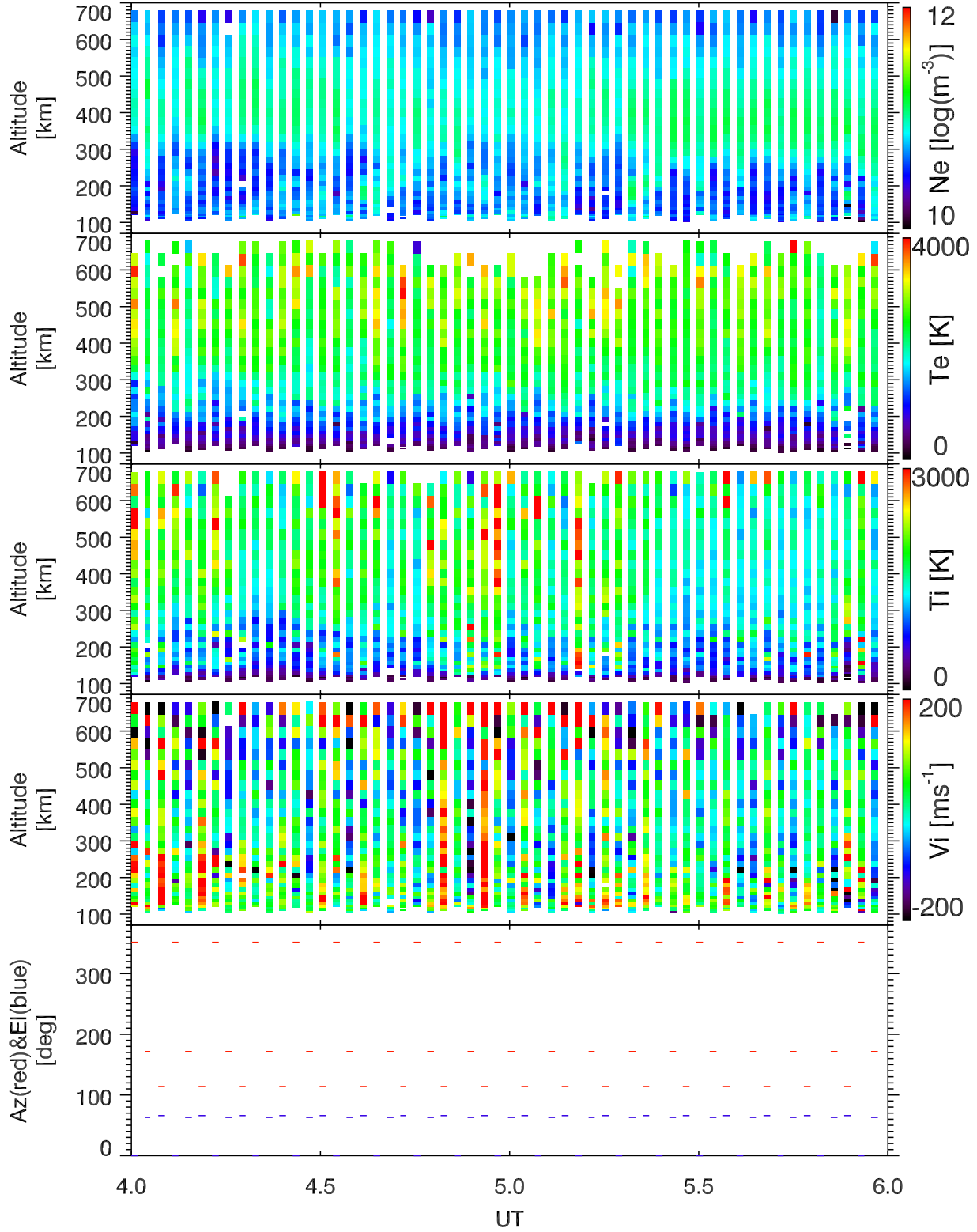
EISCAT 2002-10-29_04_06UT_tau0_ant@32m.
