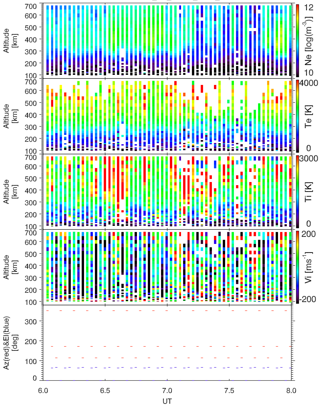
EISCAT 2002-11-02_06_08UT_tau0_ant@32m.
