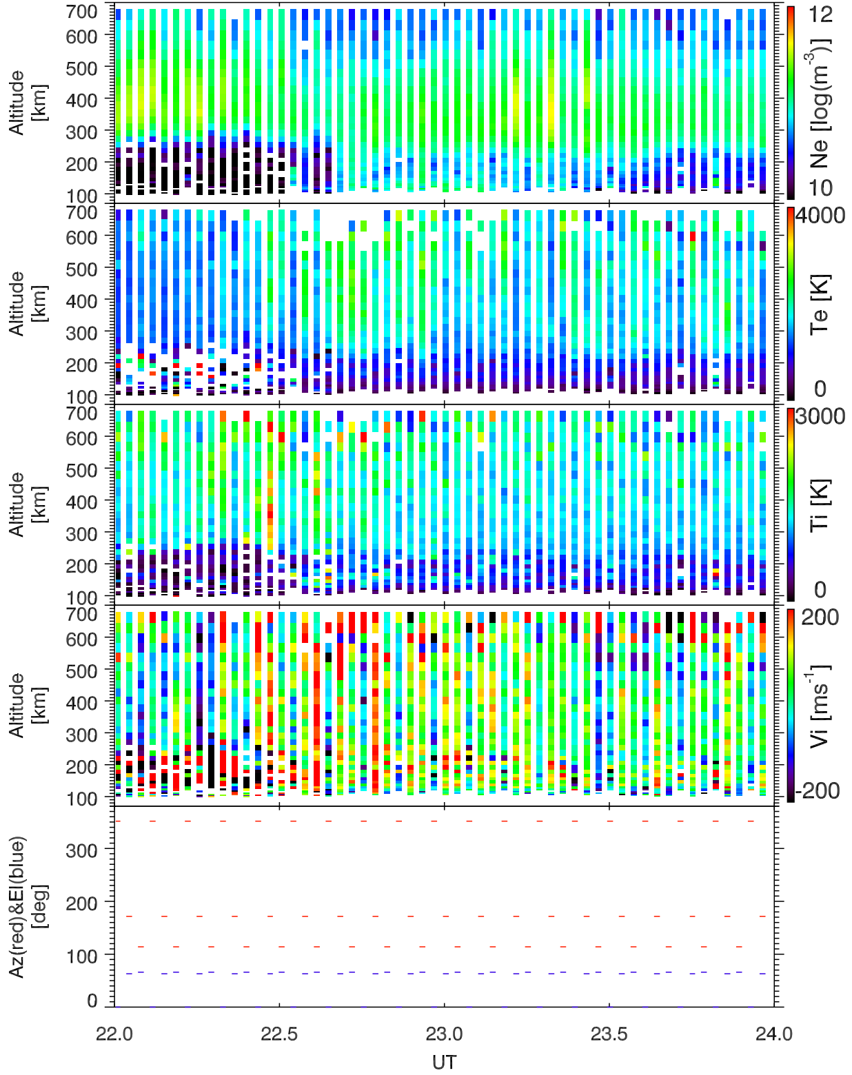
EISCAT 2002-11-11_22_24UT_tau0_ant@32m.
