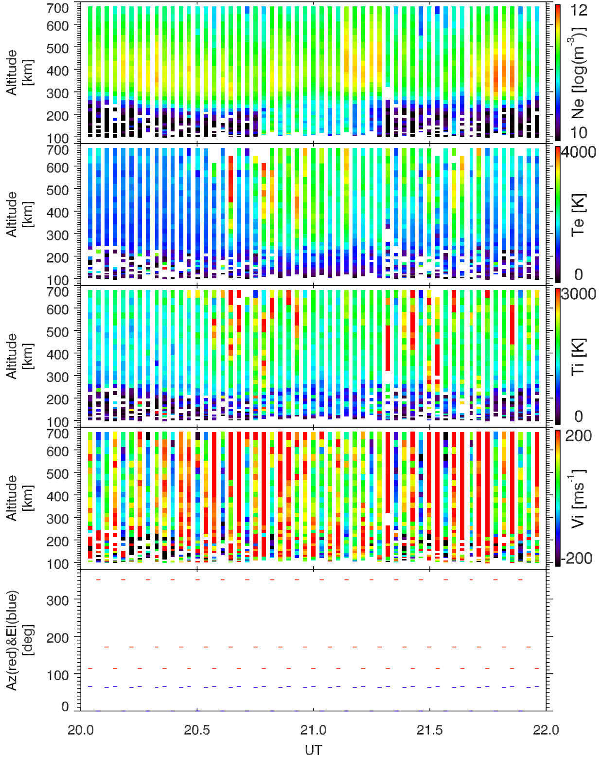
EISCAT 2002-11-12_20_22UT_tau0_ant@32m.
