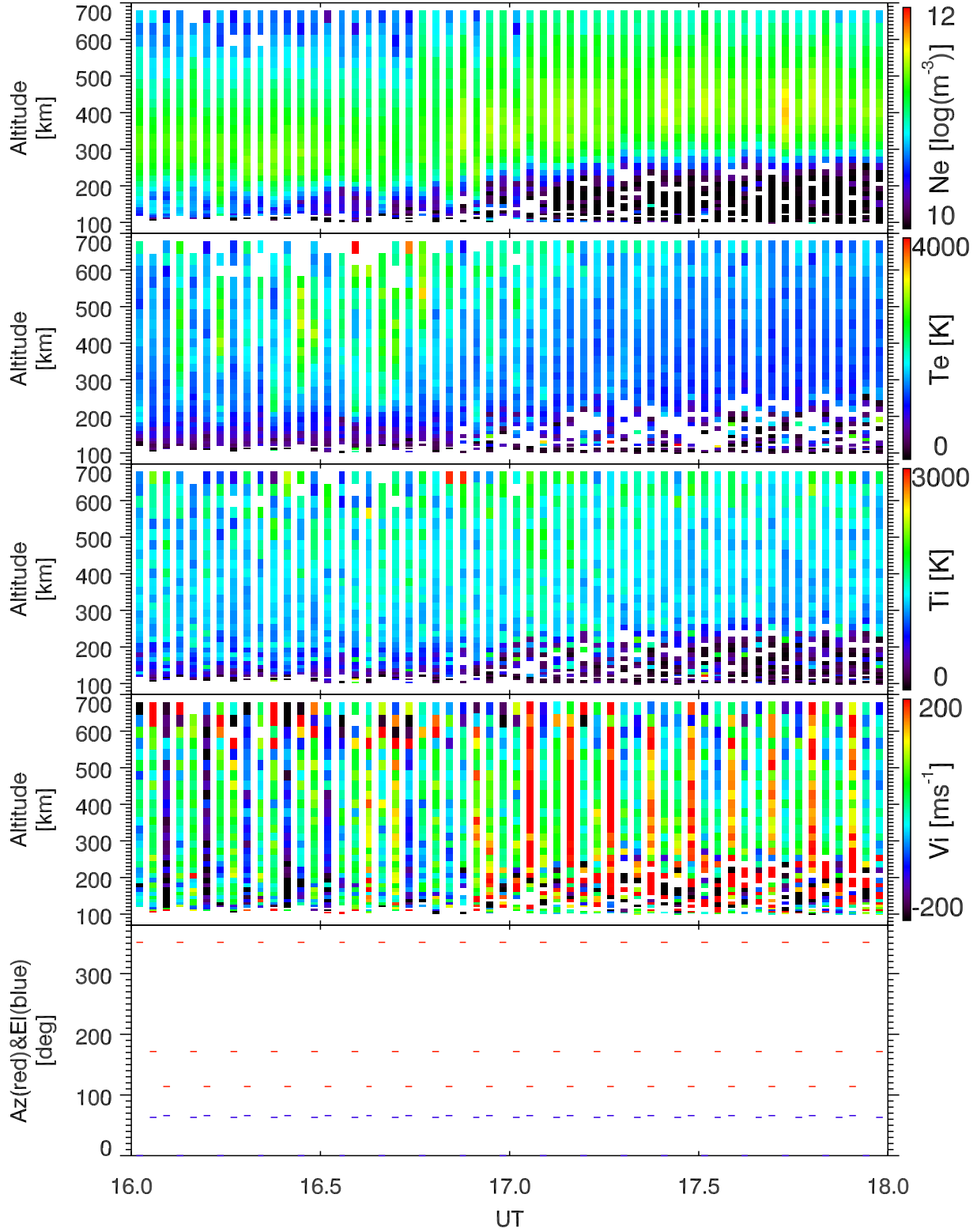
EISCAT 2002-11-14_16_18UT_tau0_ant@32m.
