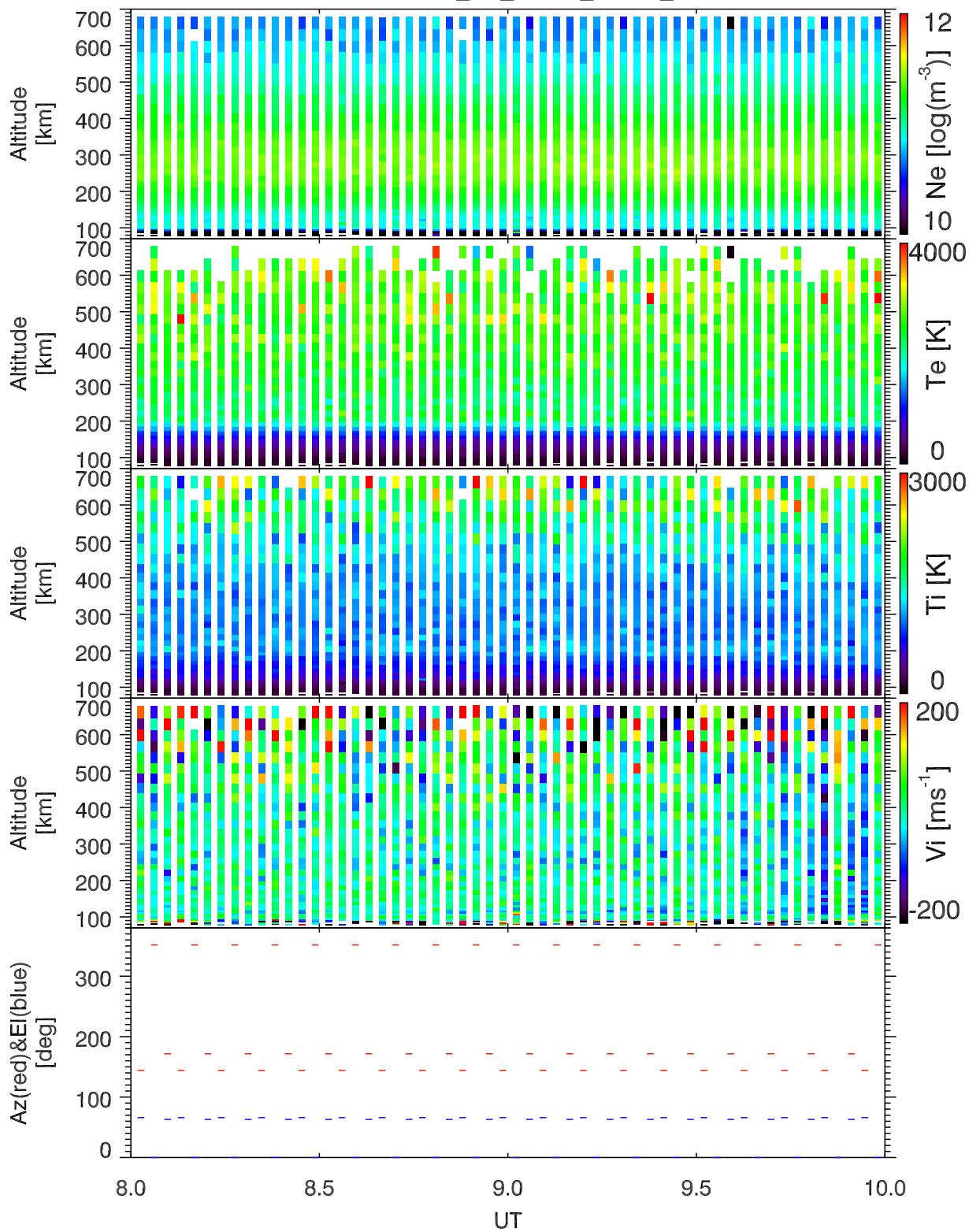
EISCAT 2004-06-05_08_10UT_steffe_ant@32m.
