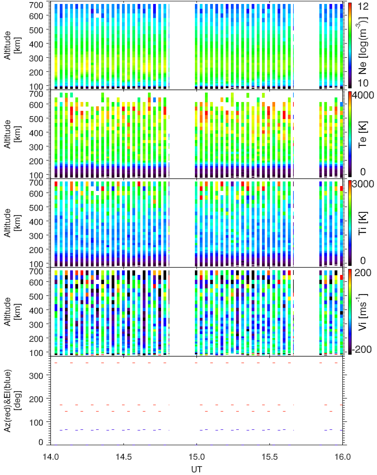
EISCAT 2004-06-07_14_16UT_steffe_ant@32m.
