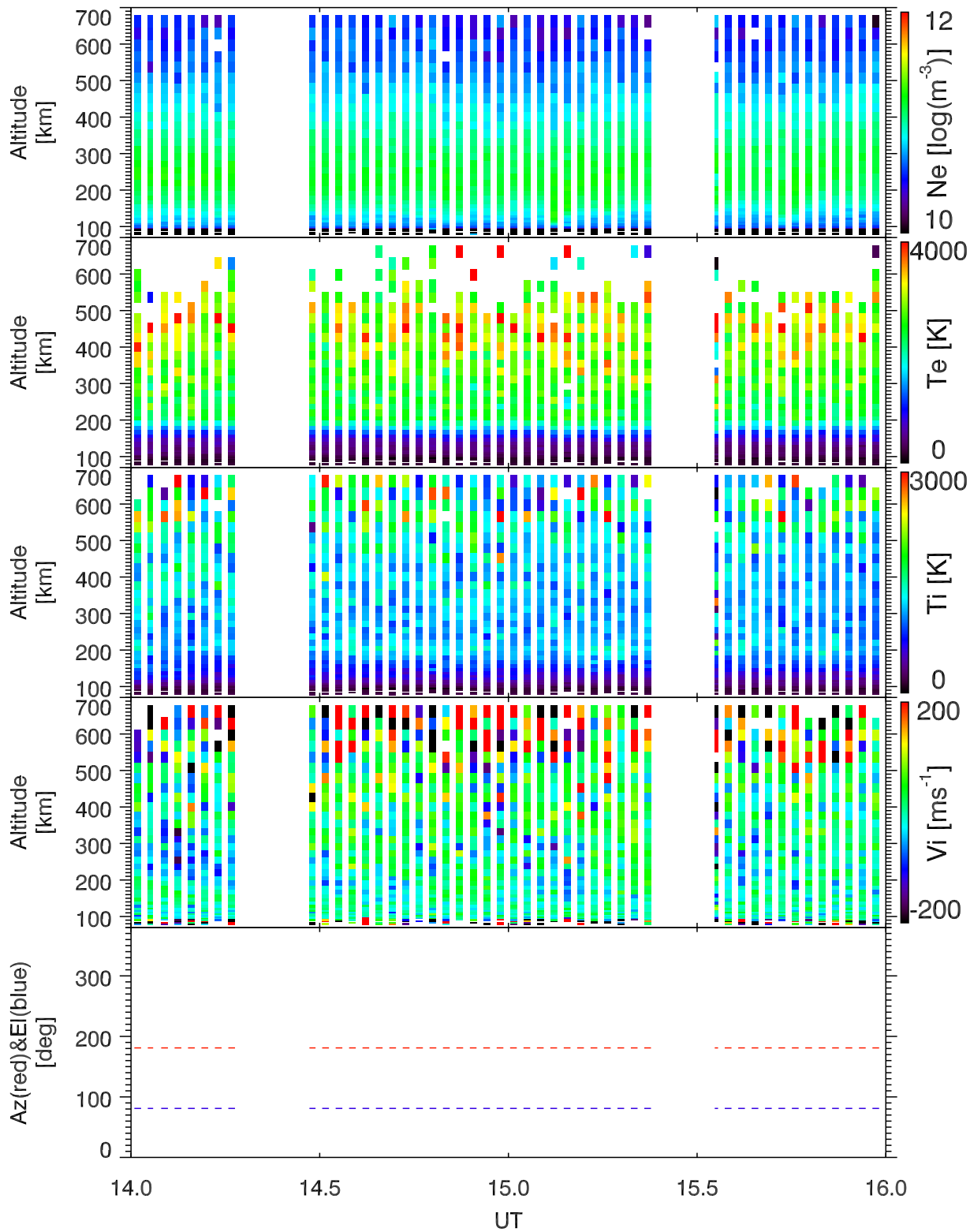
EISCAT 2004-06-08_14_16UT_steffe_ant@42m.
