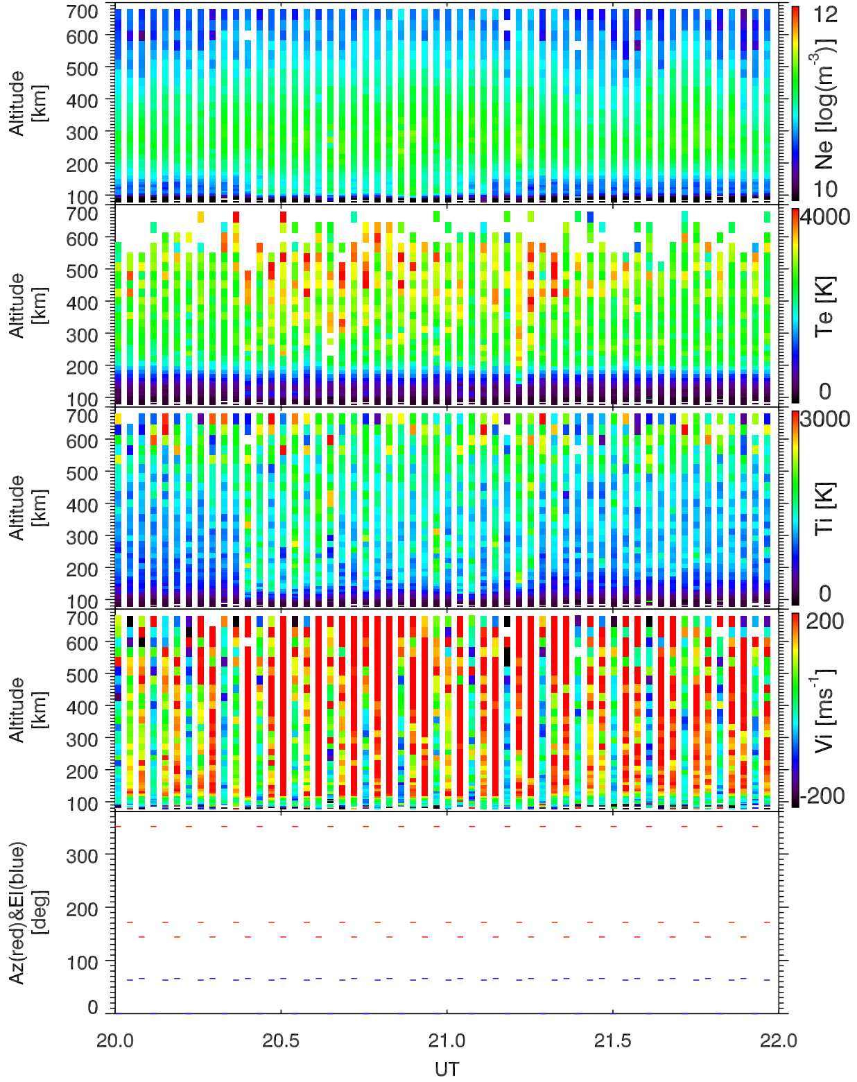
EISCAT 2004-06-10_20_22UT_steffe_ant@32m.
