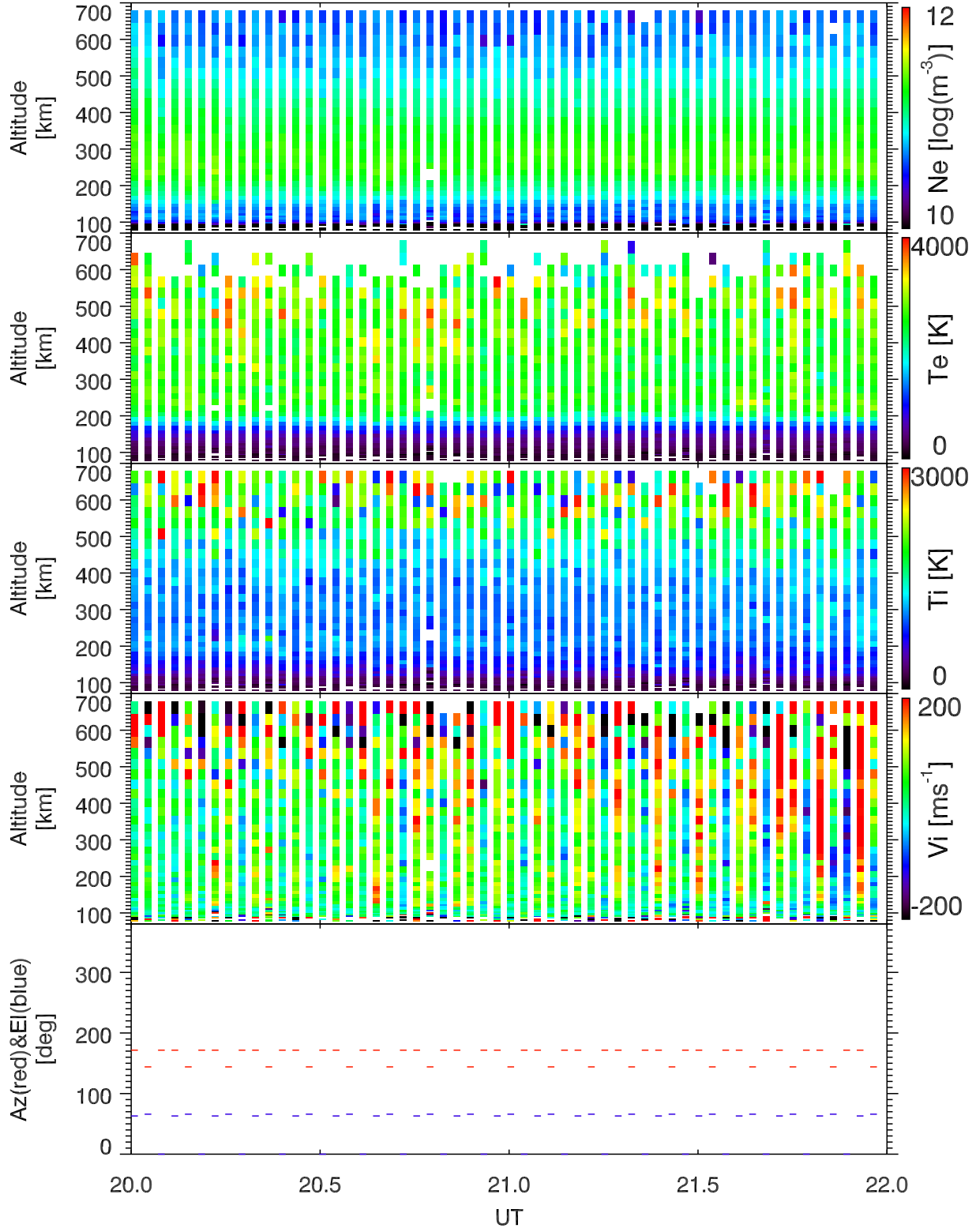
EISCAT 2004-06-13_20_22UT_steffe_ant@32m.
