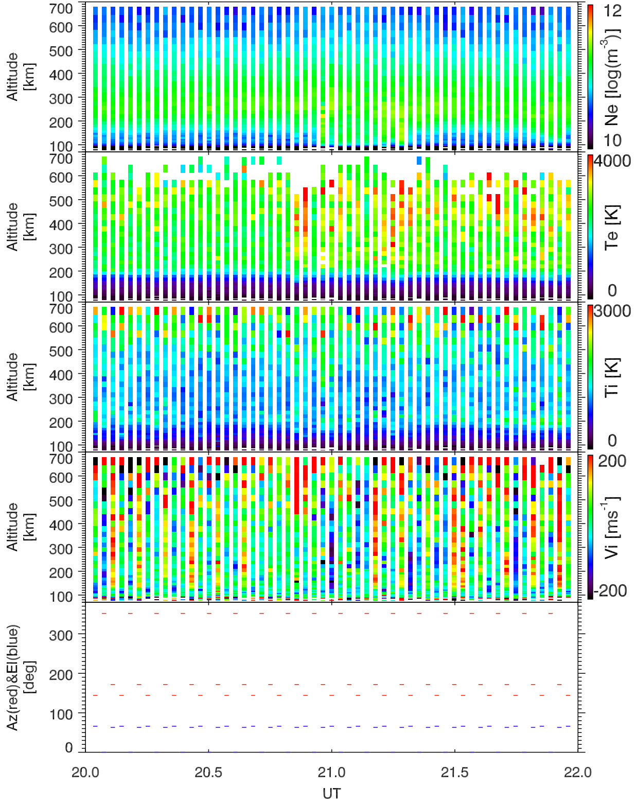
EISCAT 2005-06-14_20_22UT_steffe_ant@32m.
