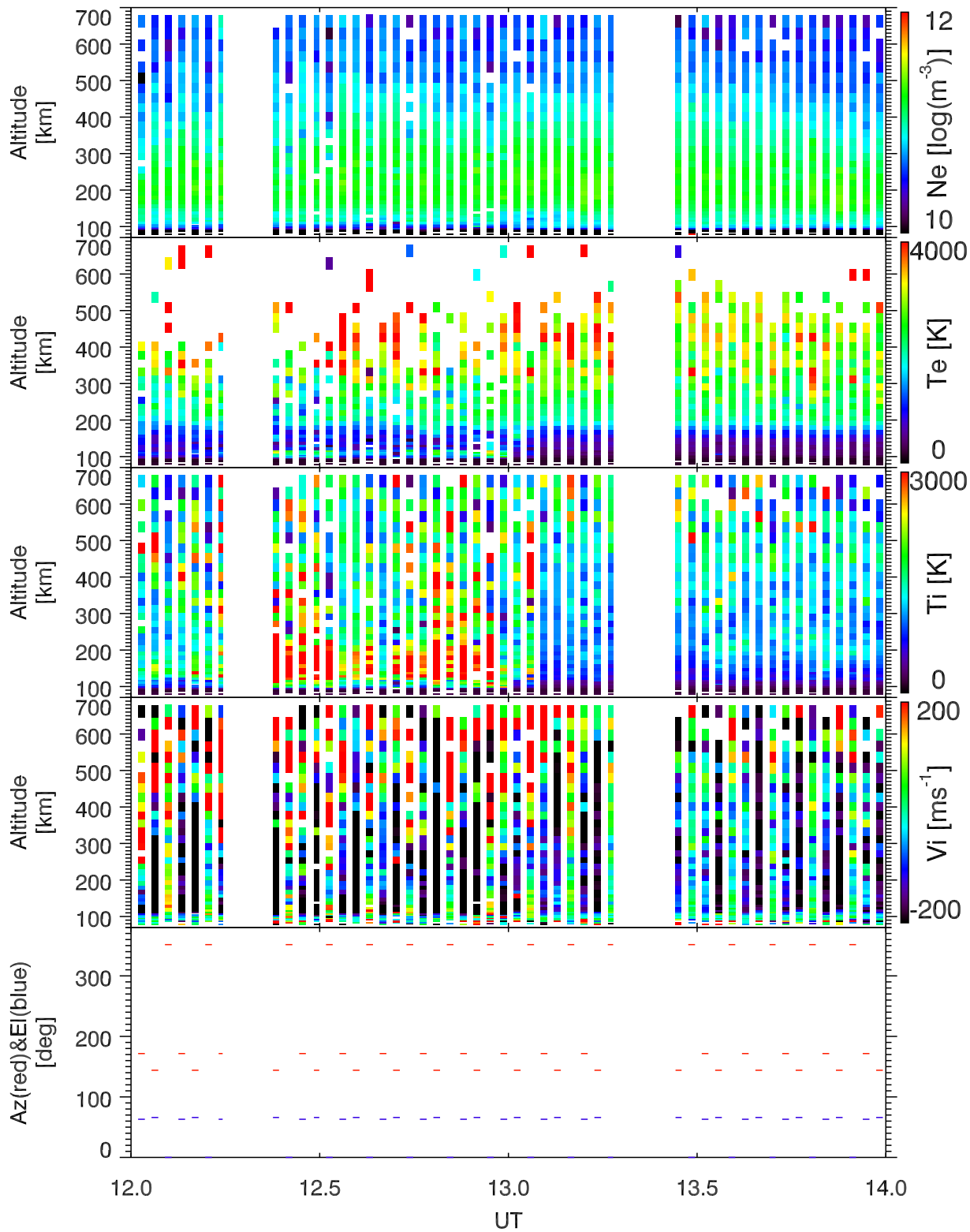
EISCAT 2005-06-16_12_14UT_steffe_ant@32m.
