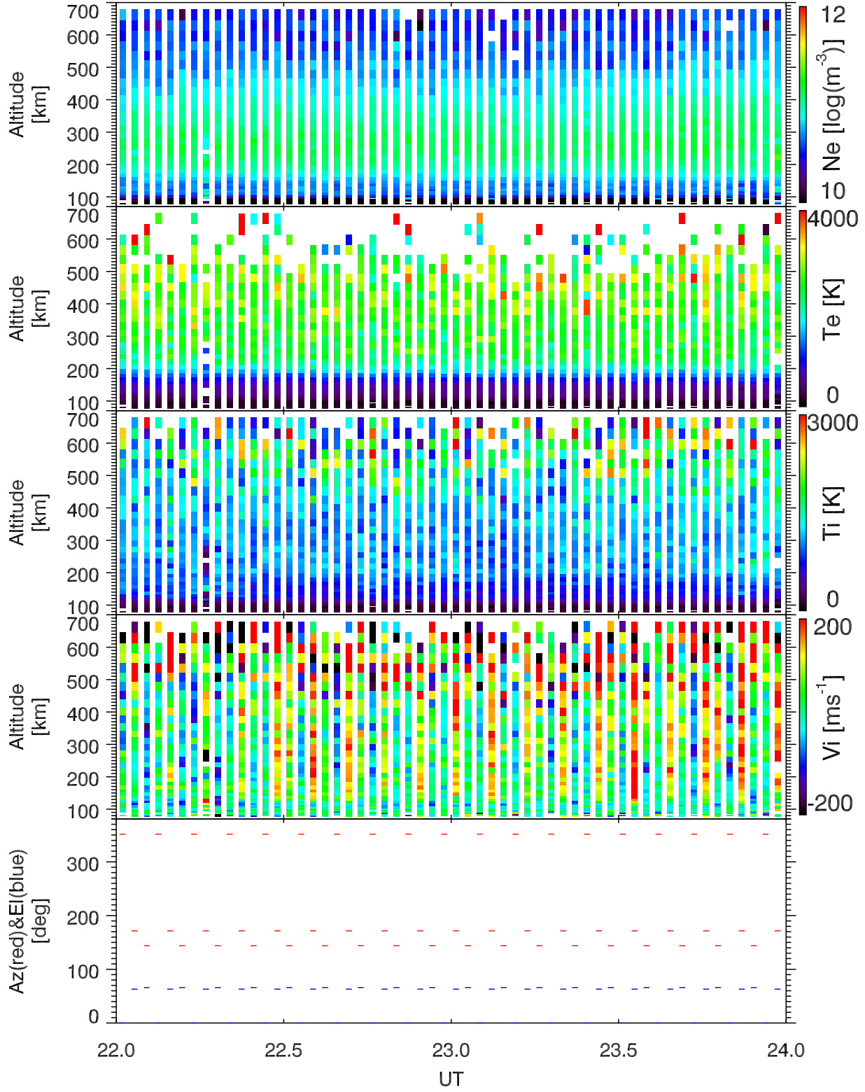
EISCAT 2005-06-16_22_24UT_steffe_ant@32m.
