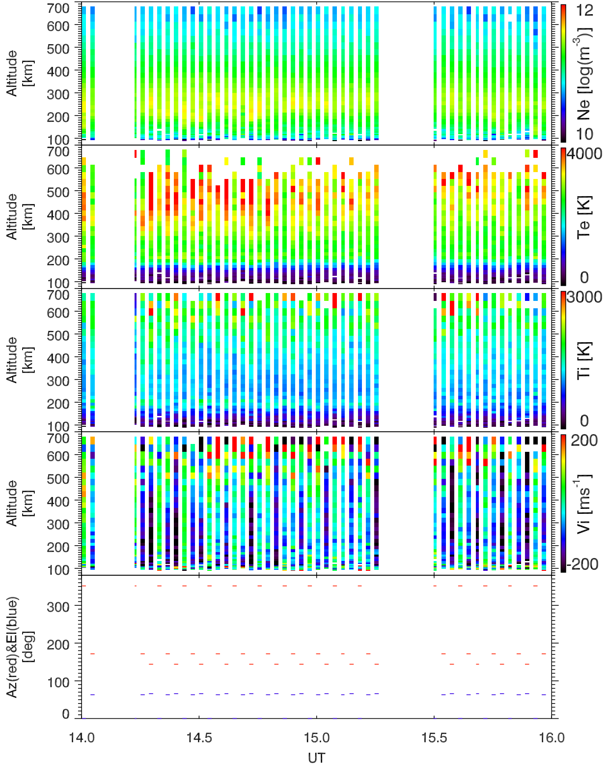
EISCAT 2005-07-01_14_16UT_tau0_ant@32m.
