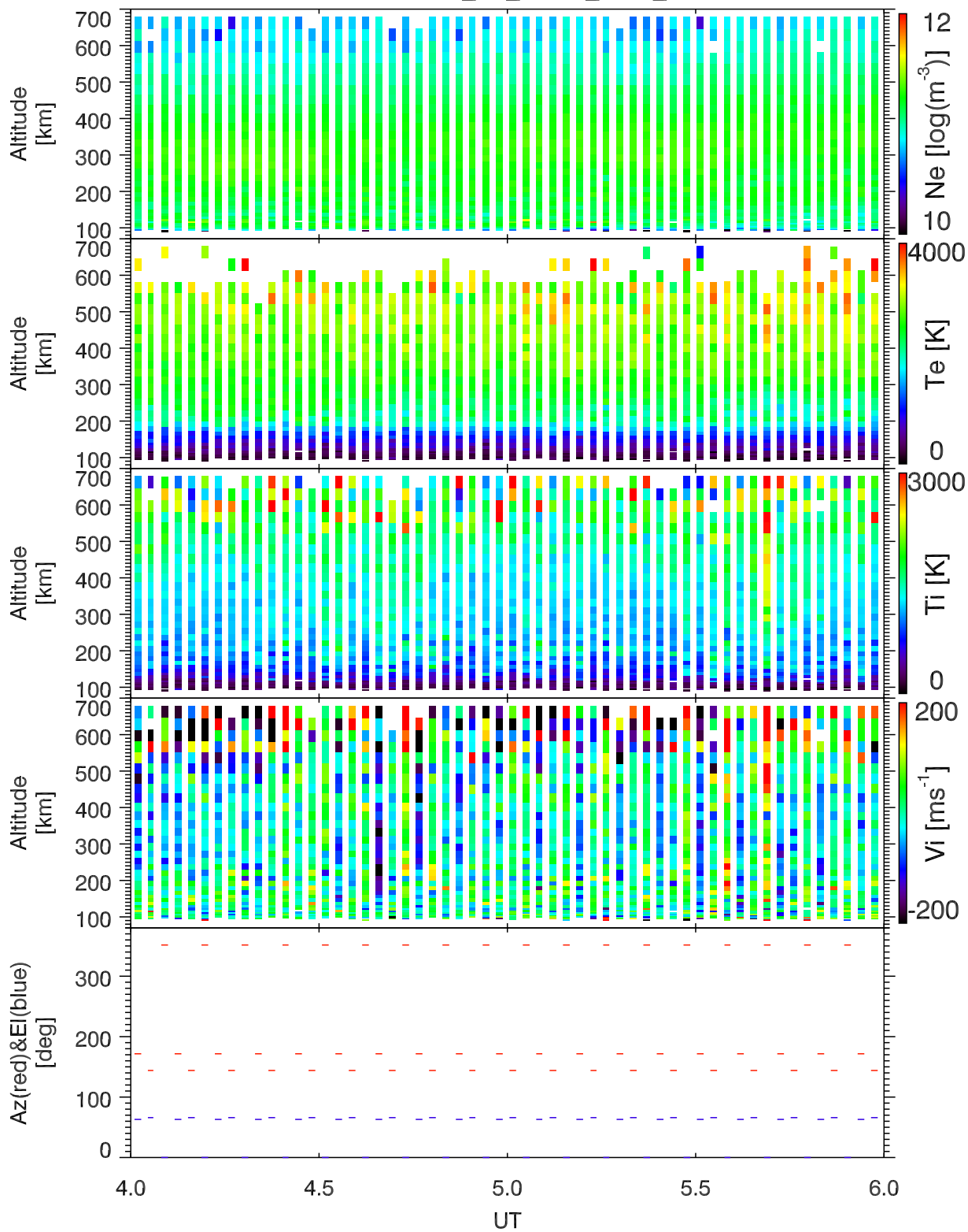
EISCAT 2005-07-02_04_06UT_tau0_ant@32m.
