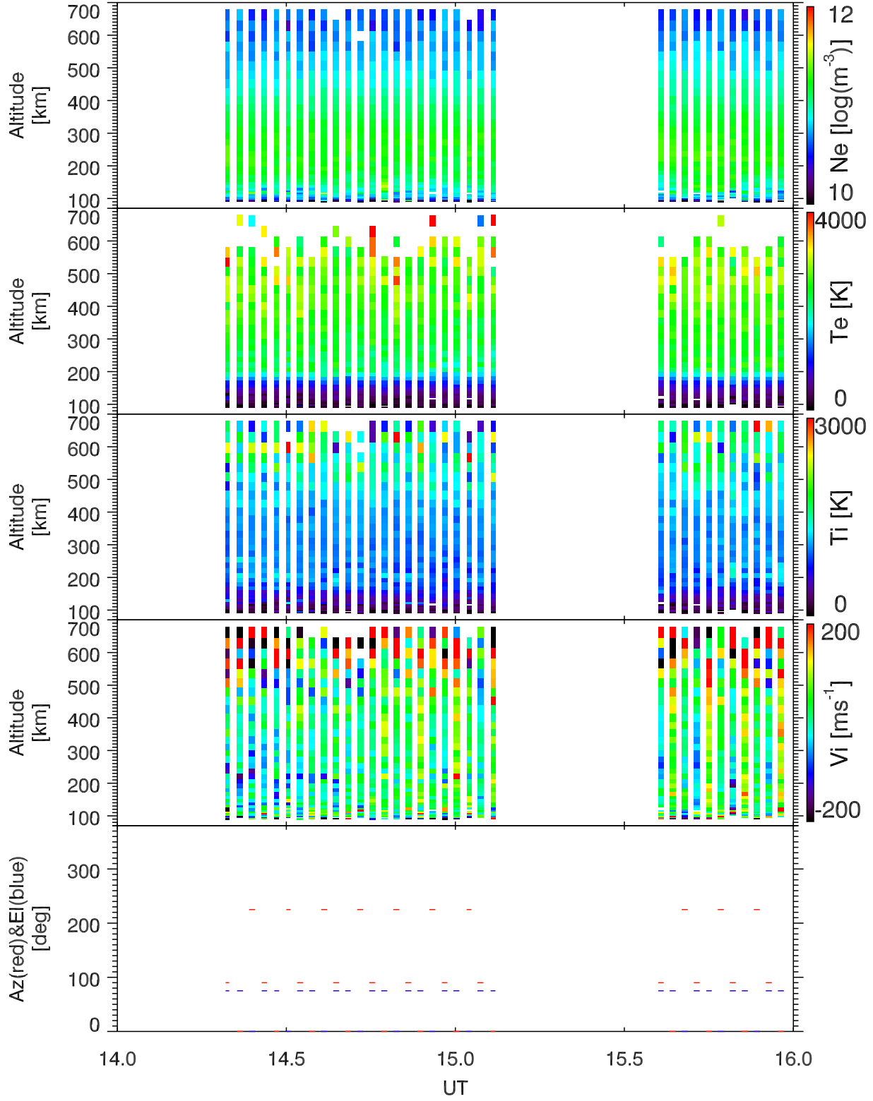
EISCAT 2005-07-22_14_16UT_tau0_ant@32m.
